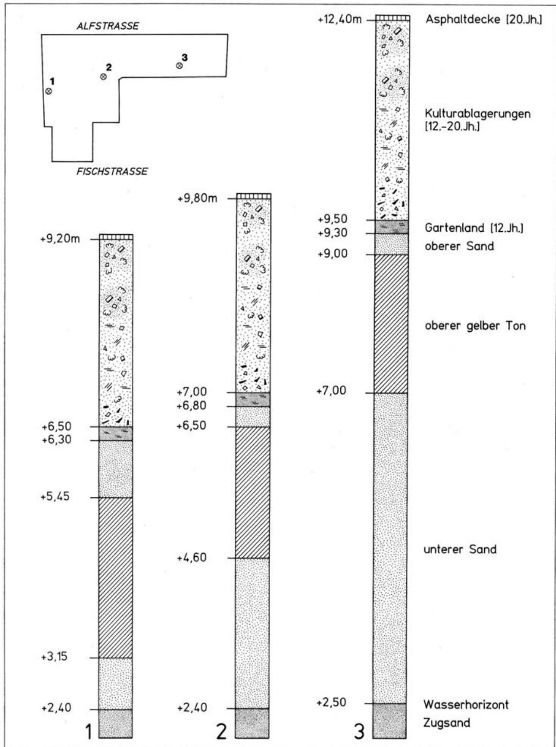
Abb. 13 Hansestadt Lübeck, Alfstraße-Fischstraße-Schüsselbuden. Rekonstruierte Profile zum Aufbau des geologischen Untergrundes und der Kulturablagerungen, erstellt nach den Profilzeichnungen und Bohrungen (1: Abschnitte 13, 26, 38 u. 45; 2: Abschnitte 50 u. 71 sowie 3: Abschnitte 29 u. 51).
