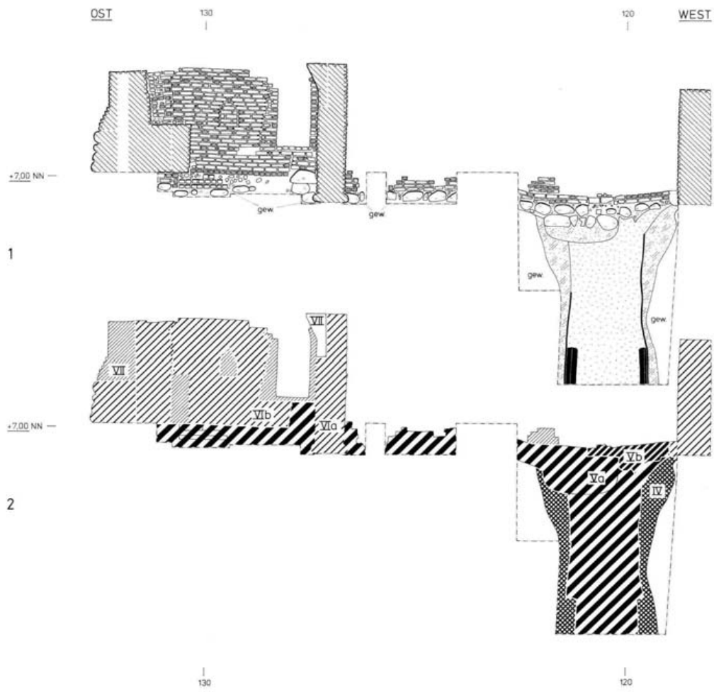
Abb. 106 Hansestadt Lübeck, Alfstraße-Fischstraße-Schüsselbuden. Alfstraße 5, Siedlungsperioden IV-VII, Mauerwerksansicht M 2, Brunnen 8, Südwand Haus 22 und jüngeres Mauerwerk. 1 Steingerechtes Aufmaß. 2 Periodisierung.
