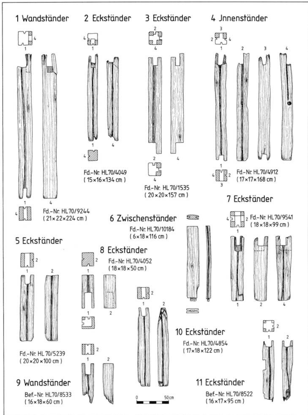
Abb. 98 Hansestadt Lübeck, Alfstraße-Fischstraße-Schüsselbuden. In verworfener Lage erfaßte Ständer in Stabbauweise. 1 Wandständer (Alfstr. 7, Per. Vb). 2 Eckständer (Alfstraße 11, Per. VIa). 3 Eckständer (Fischstraße 12/14, Per. IV). 4 Innenständer (Alfstraße 11, Per. Vb). 5 Eckständer (Alfstraße 9, Per. IV). 6 Zwischenständer (Fischstraße 12, Per. IV). 7 Eckständer (Alfstraße 9, Per. IV). 8 Eckständer (Alfstraße 11, Per. Va). 9 Wandständer (Alfstraße 9, Per. Vb). 10 Eckständer (Alfstraße 11, Per. Vb). 11 Eckständer (Alfstraße 9, Per. IV).
