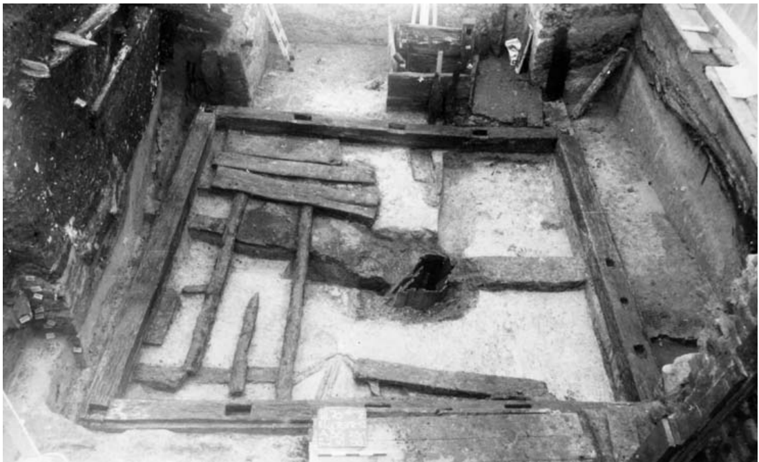
Abb. 45 Hansestadt Lübeck, Alfstraße-Fischstraße-Schüsselbuden. Fischstraße 12, Siedlungsperiode IV, Haus 8, Schwellenkranz sowie Reste des Holzfußbodens, hinten Brunnen 3 mit "Drainagerinne", mittig Brunnen 4, von Westen (Neg.-Nr. 17650).
