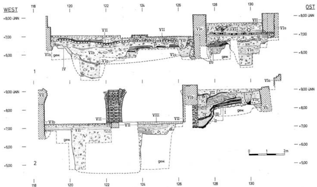
Abb. 108 Hansestadt Lübeck, Alfstraße-Fischstraße-Schüsselbuden. 1 Hangprofil PIII, Rekonstruktion der Hofstelle 1 mit den Häusern 2 u. 3, Brunnen 2 und Arbeitsgruben 2 u. 3 sowie der Hofstelle 3 mit den Häusern 5 u. 6 und Vorratsgrube 3 (Lage vgl. Abb. 27). 2 Hangprofil PIV, Rekonstruktion des Stadthofes 1 mit den Häusern 7 u. 8, des Stadthofes 2 mit den Häusern 11 u. 12, des Stadthofes 3 mit Haus 14 sowie der Hofstelle 3 mit den Häusern 5, 19 u. 20 und Brunnen 8 (Lage vgl. Abb. 42).
