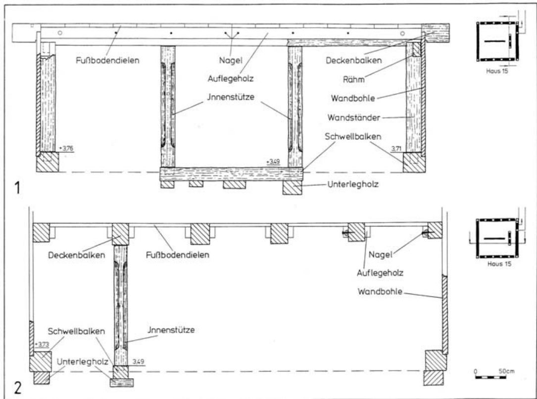
Abb. 62 Hansestadt Lübeck, Alfstraße-Fischstraße-Schüsselbuden. Alfstraße 11, Siedlungsperiode IV, Haus 15, Bauegefüge Kellergeschoß. 1 Nordwärtschnitt. 2 Ostwärtschnitt.
