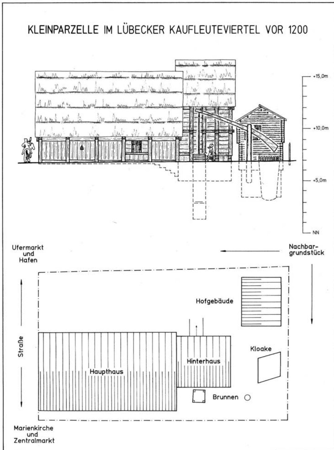
Abb. 87 Hansestadt Lübeck, Alfstraße-Fischstraße-Schüsselbuden. Fischstraße 12-14, Siedlungsperiode IV, Stadthof 1. Rekonstruktion der aufgehenden Bebauung eines Stadthofes, Ansicht und Grundriß.
