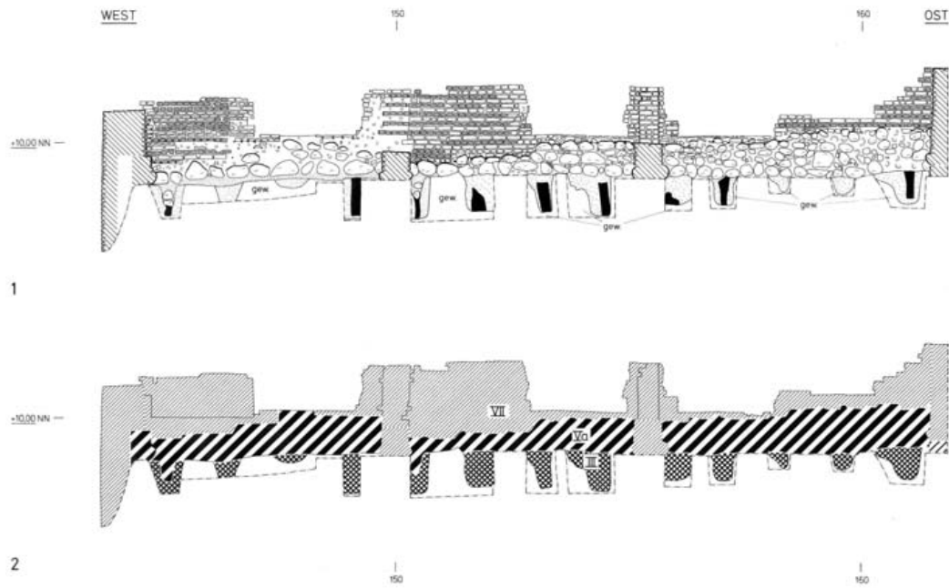
Abb. 104 Hansestadt Lübeck, Alfstraße-Fischstraße-Schüsselbuden. Schüsselbuden 6, Siedlungsperioden III, Va u. VII, Mauerwerksansicht M 4, nördliche Pfostengrubenzeile Haus 5, Nordwand Haus 21 sowie jüngeres Mauerwerk. 1 Steingerechtes Aufmaß. 2 Periodisierung.
