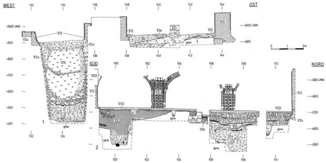
Abb. 110 Hansestadt Lübeck, Alfstraße-Fischstraße-Schüsselbuden. 1 Nordprofil P 1, Teil 2, Alfstraße 1 (Achsen 133-144). 2 Westprofil P 11, Alfstraße 5 (Achsen 99-111, Lage vgl. Abb. 11).
