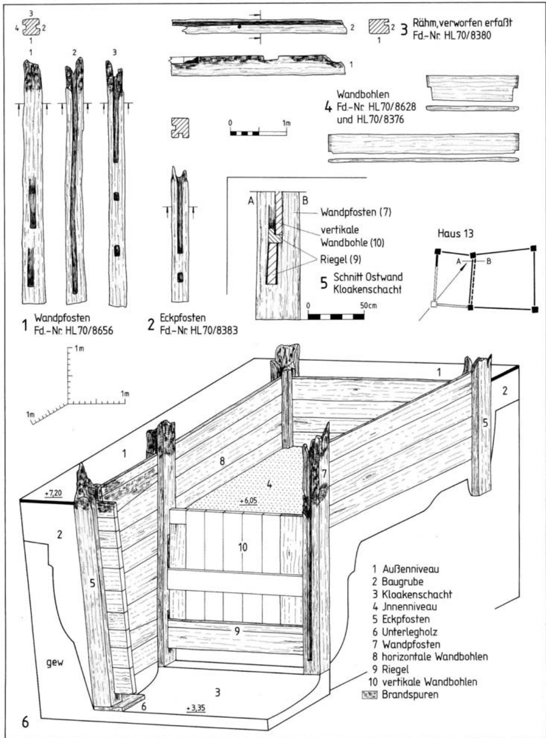
Abb. 54 Hansestadt Lübeck, Alfstraße-Fischstraße-Schüsselbuden. Fischstraße 10, Siedlungsperiode IV, Haus 13. 1 u. 2 Gerüstpfosten. 3 Rähm. 4 Wandbohlen. 5 Schnitt durch Innenwand. 6 Isometrie der in situ erfaßten Konstruktion.
