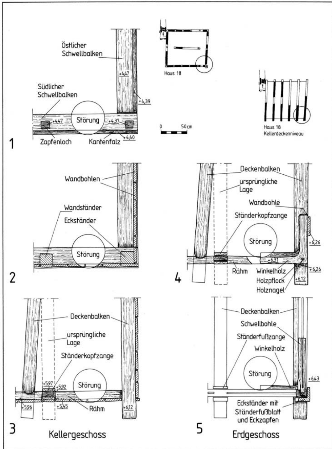
Abb. 73 Hansestadt Lübeck, Alfstraße-Fischstraße-Schüsselbuden. Alfstraße 7-9, Siedlungsperiode IV, Haus 18, Südostecke, Bauefüge Kellergeschoß: 1 Aufsicht Schwellenkranz. 2 Schnitt Wandständer u. Wandbohlen. 3 Aufsicht Ständerkopf, Rähm u. Deckenbalken. Bauefüge Erdgeschoß: 4 Aufsicht Winkelholz mit Holznagel und seitlichem Holzpflöck über Kellerdeckenbalken und Rähm. 5 Aufsicht Schwellbohlen und Schnitt Eckständerfuß über Winkelholz.
