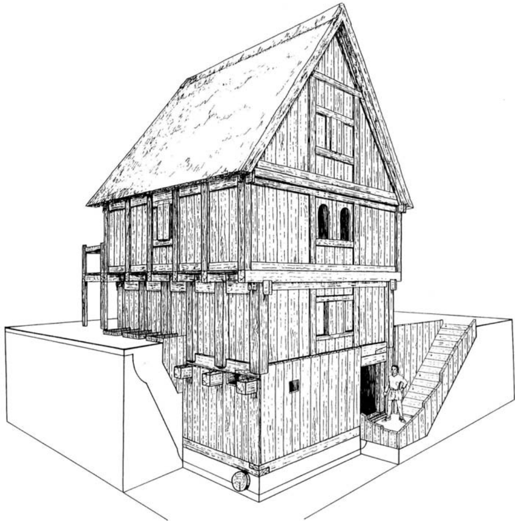
Abb. 97 Hansestadt Lübeck, Alfstraße-Fischstraße-Schüsselbuden. Rekonstruktion der aufgehenden Konstruktion über dem Keller Haus 15 als dreigeschossiger Stockwerksbau, ergänzt durch den Befund Haus 18 sowie verworfener Bauhölzer.
