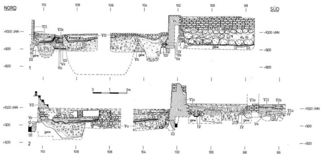
Abb. 121 Hansestadt Lübeck, Alfstraße-Fischstraße-Schüsselbuden. 1 Ostprofil P 12, Schüsselbuden 6-8 (Achsen 98-110). 2 Ostprofil P 13, Schüsselbuden 6-8 (Achsen 96-111, Lage vgl. Abb. 11).
