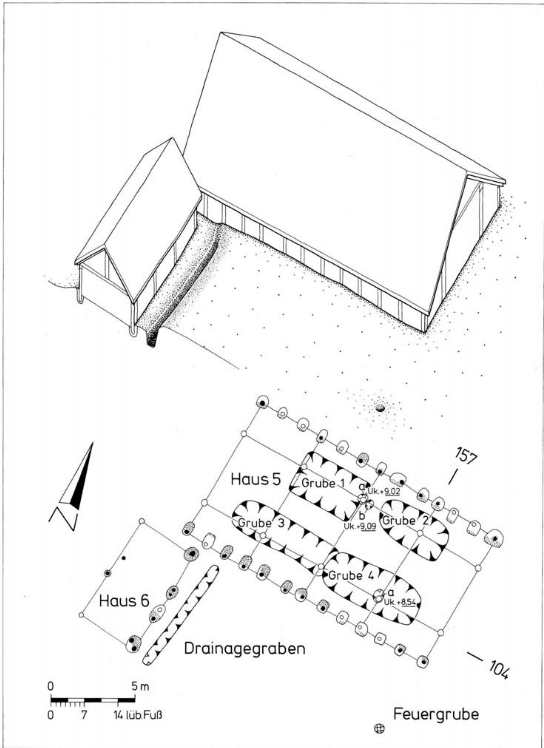
Abb. 39 Hansestadt Lübeck, Alfstraße-Fischstraße-Schüsselbuden. Schüsselbuden 6-8, Siedlungsperiode III, Haus 5 mit jüngeren Gruben 1-4 und Haus 6, isometrische Skizze zur Rekonstruktion der Hausbefunde.
