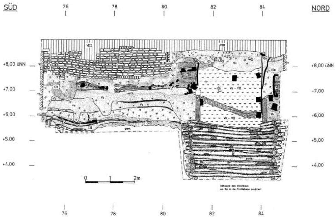
Abb. 115 Hansestadt Lübeck, Alfstraße-Fischstraße-Schüsselbuden. Westprofil P 7, Fischstraße 14 (Achsen 75-85, Lage vgl. Abb. 11).
