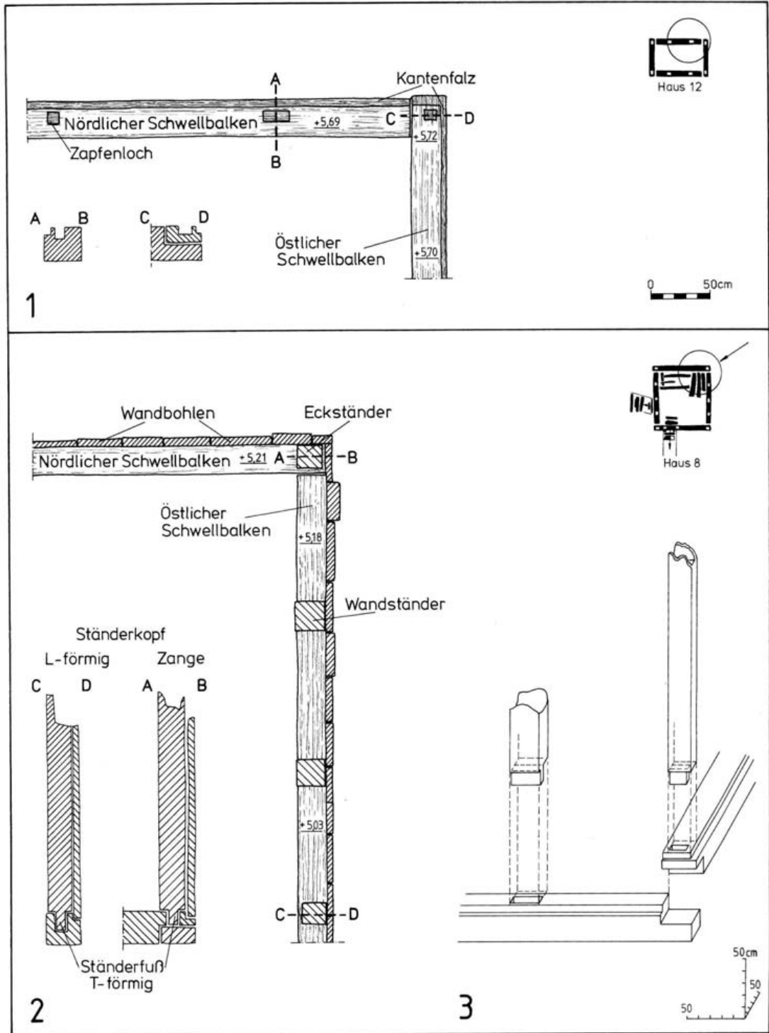
Abb. 46 Hansestadt Lübeck, Alfstraße-Fischstraße-Schüsselbuden. Fischstraße 10-12, Siedlungsperiode IV, Häuser 8 und 10, Baugefüge der Kellergeschosse. 1 Haus 10, Schwellenkranz, Aufsicht und Schnitte. 2 Haus 8, Schwellenkranz u. Wandständer, Aufsicht und Schnitte. 3 Haus 8, Isometrie der Eckkonstruktion.
