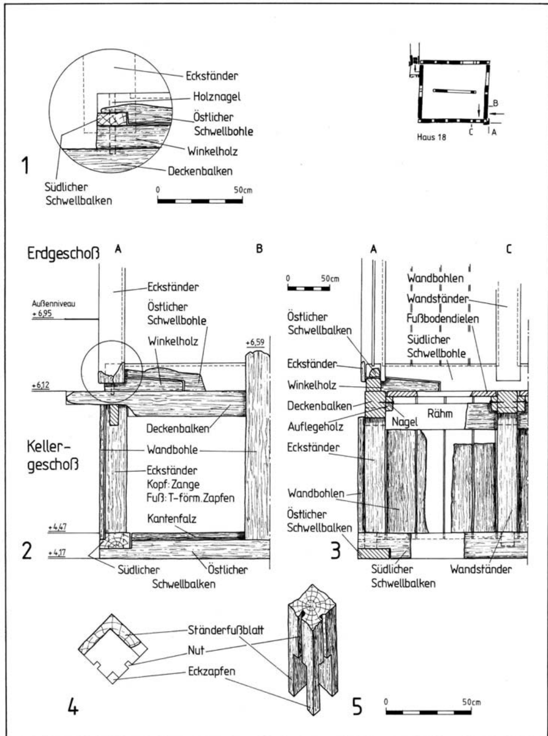
Abb. 75 Hansestadt Lübeck, Alfstraße-Fischstraße-Schüsselbuden. Alfstraße 7-9, Siedlungsperiode IV, Haus 18. 1 Erdgeschoß Gefügeknoten, 2 Außenansicht Ostwand. 3 Innenansicht Südwand. 4 Ansicht Ständerfuß des rekonstruierten Eckständers. 5 verworfener Eckständer mit Ständerfußblatt.
