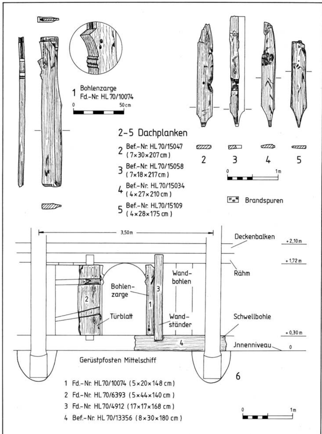
Abb. 95 Hansestadt Lübeck, Alfstraße-Fischstraße-Schüsselbuden. In verworfener Lage erfaßte Bauhölzer. 1 Bohlenzarge (Fischstraße 12, Periode IV, HL 70/10074). 2-5 Dachplanken (Fischstraße 12, Periode IV, Bef.-Nr. HL 70/15047, HL 70/15058, HL 70/15034, HL 70/15109). 6 Rekonstruktion eines Wandausschnitts mit Türöffnung anhand verworfener Bauhölzer.
