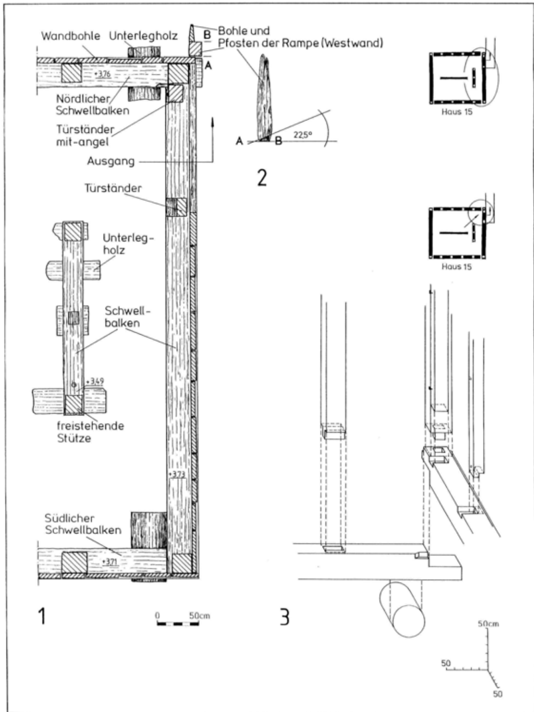
Abb. 58 Hansestadt Lübeck, Alfstraße-Fischstraße-Schüsselbuden. Alfstraße 11, Siedlungsperiode IV, Haus 15, Bauefüge Kellergeschoß. 1 Aufsicht Schwellenkranz mit Türausgang, Rampenanlage und Schwellbalken der freistehenden Stützen. 2 Wandpfosten der Rampenanlage. 3 Isometrie der nordöstlichen Eckkonstruktion mit Türständern.
