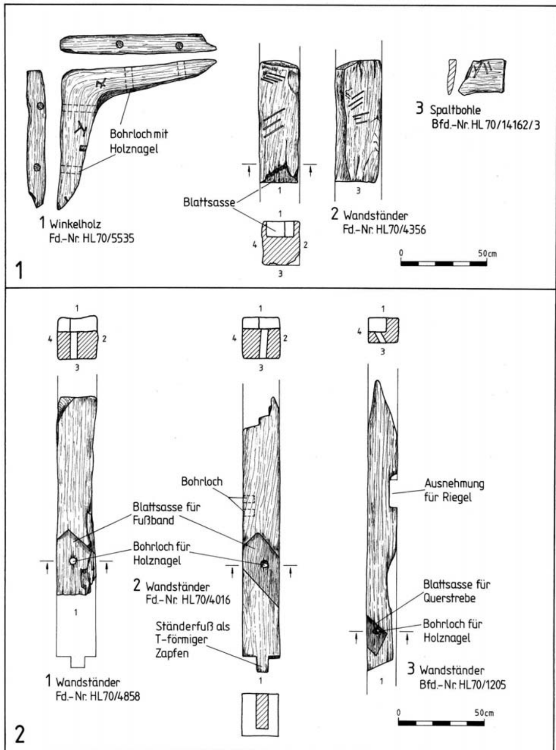
Abb. 99 Hansestadt Lübeck, Alfstraße-Fischstraße-Schüsselbuden. 1 In verwerfener Lage erfaßte Bauhölzer mit Strichmarkierungen. 1.1 Winkelholz (Alfstraße 11, Per. V). 1.2 Wandständer (Alfstraße 9, Per. VI). 1.3 Spaltbohle (Alfstraße 7, Per. V). 2 In verwerfener Lage erfaßte Ständer mit Blattsasse. 2.1 Wandständer (Alfstraße 11, Per. Vb). 2.2 Wandständer (Alfstraße 11, Per. Vb). 2.3 Wandständer (Fischstraße 14, Per. Vb).
