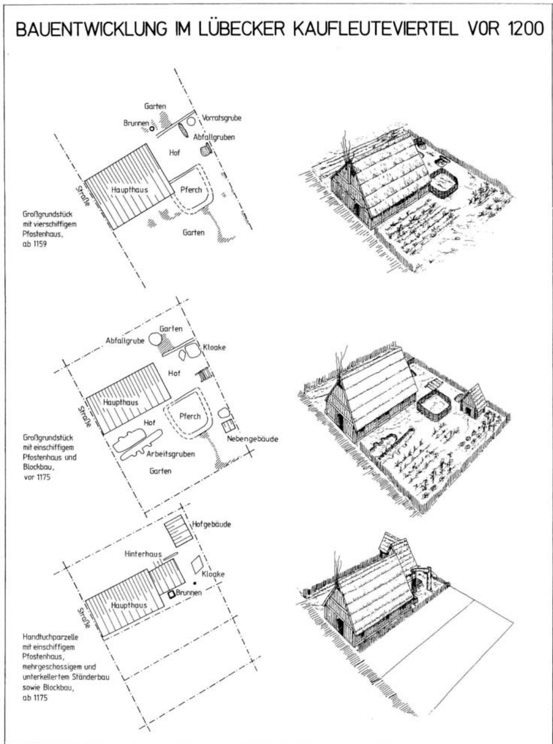
Abb. 88 Hansestadt Lübeck, Alfstraße-Fischstraße-Schüsselbuden. Fischstraße 8-14, Siedlungsperioden II-IV, Hofstelle 1 u. Stadthöfe 1-3. Rekonstruktion der Grundstücksteilung und baulichen Entwicklung einer geräumigen Hofstelle und Urparzelle zu drei dicht bebauten Stadthöfen.
