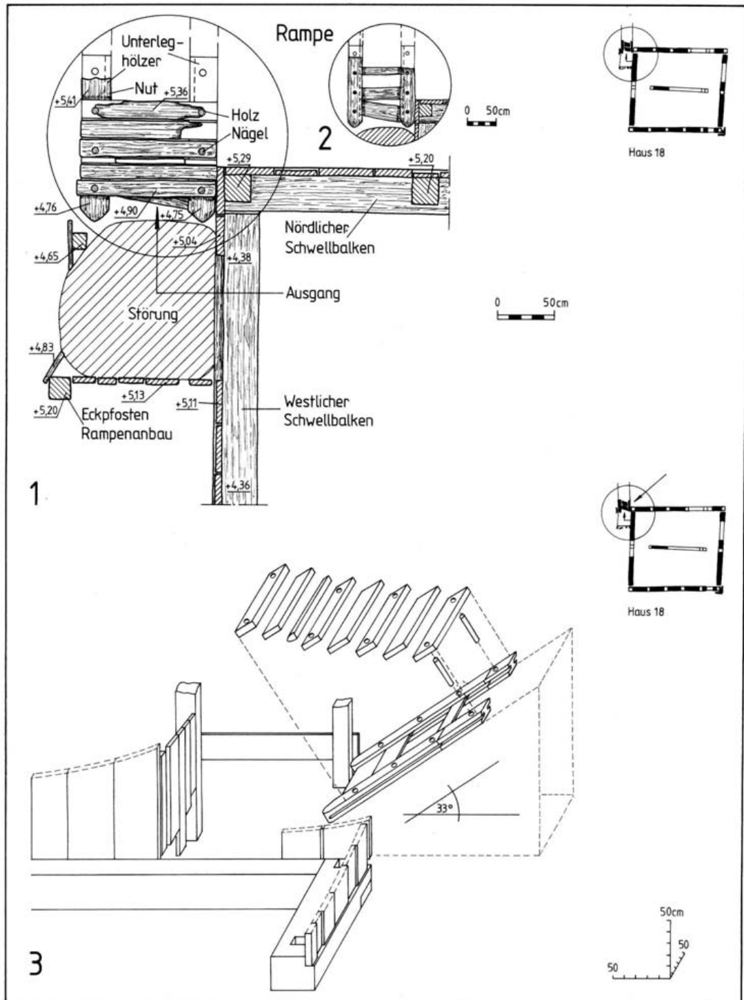
Abb. 79 Hansestadt Lübeck, Alfstraße-Fischstraße-Schüsselbuden. Alfstraße 7-9, Siedlungsperiode IV, Haus 18, Nordwestecke. 1 Aufsicht Schwellenkrans und Rampenanlage. 2 Aufsicht Rampenunterkonstruktion. 3 Isometrie Kellerausgang.
