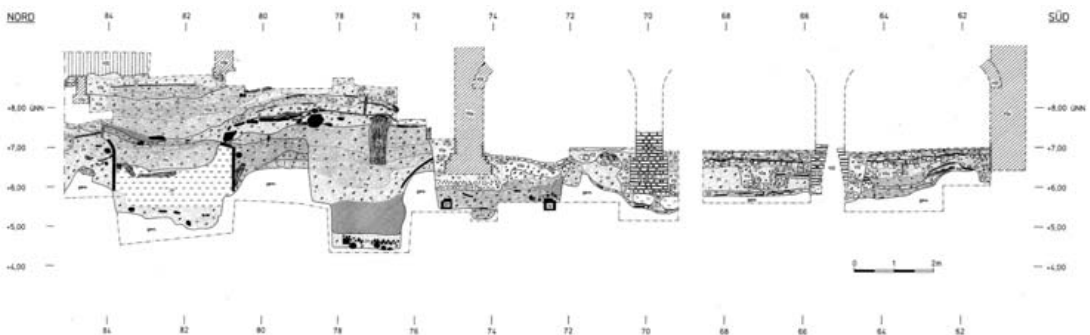
Abb. 119 Hansestadt Lübeck, Alfstraße-Fischstraße-Schüsselbuden. Ostprofil P 9, Teil 2, Fischstraße 10 (Achsen 60-85, Lage vgl. Abb. 11).
