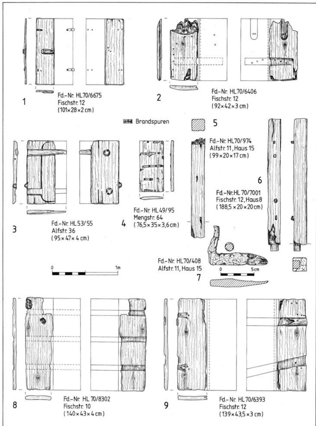
Abb. 93 Hansesstadt Lübeck, Alfstraße-Fischstraße-Schüsselbuden. In verworfener Lage erfaßte Bauhölzer. 1 Fensterladen (Fischstraße 12, Per. IV). 2 Fensterladen (Fischstraße 12, Per. V). 3 Fensterladen (Alfstraße 36, Dd. "um oder nach 1169"). 4 Fensterladen (Mengstraße 64, nach 1206). 5 Türständer mit Türangeln (Alfstraße 11, Periode IV). 6 Türständer mit Türangeln (Fischstraße 12, Per. IV). 7 Türangel (Alfstraße 11, Per. IV). 8 Türblatt (Fischstraße 10, Per. V). 9 Türblatt (Fischstraße 12, Per. V).
