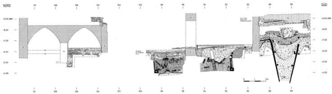
Abb. 118 Hansestadt Lübeck, Alfstraße-Fischstraße-Schüsselbuden. Ostprofil P 9, Teil 1, Alfstraße 9 (Achsen 84-109, Lage vgl. Abb. 11).
