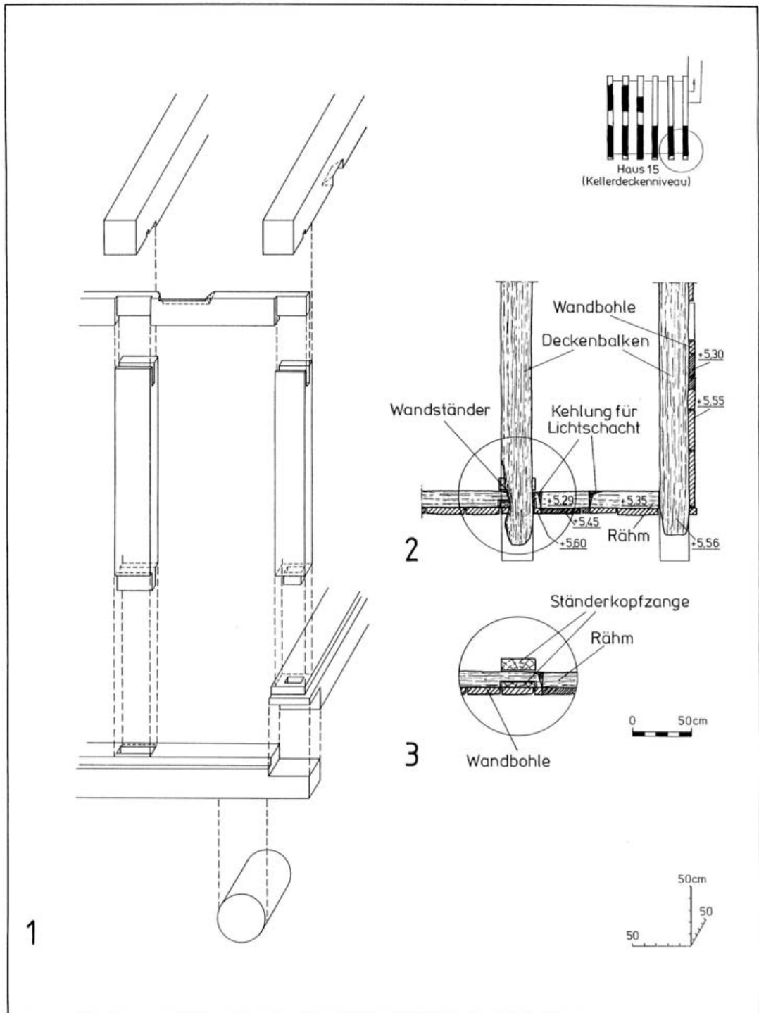
Abb. 59 Hansestadt Lübeck, Alfstraße-Fischstraße-Schüsselbuden. Alfstraße 11, Siedlungsperiode IV, Haus 15, Bauegefüge Kellergeschoß. 1 Isometrie der südöstlichen Eckkonstruktion mit Rähm und Deckenbalken. 2 Aufsicht Deckenbalkenniveau. 3 Aufsicht oberer Wandabschluß mit Ständerkopfzangen und Rähm.
