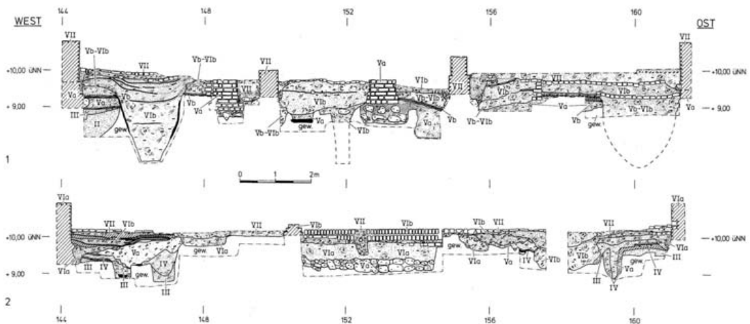
Abb. 111 Hansestadt Lübeck, Alfstraße-Fischstraße-Schüsselbuden. 1 Nordprofil P 1, Teil 3, Schüsselbuden 6 (Achsen 144-161). 2 Nordprofil P 2, Teil Schüsselbuden 8 (Achsen 144-161, Lage vgl. Abb. 11).
