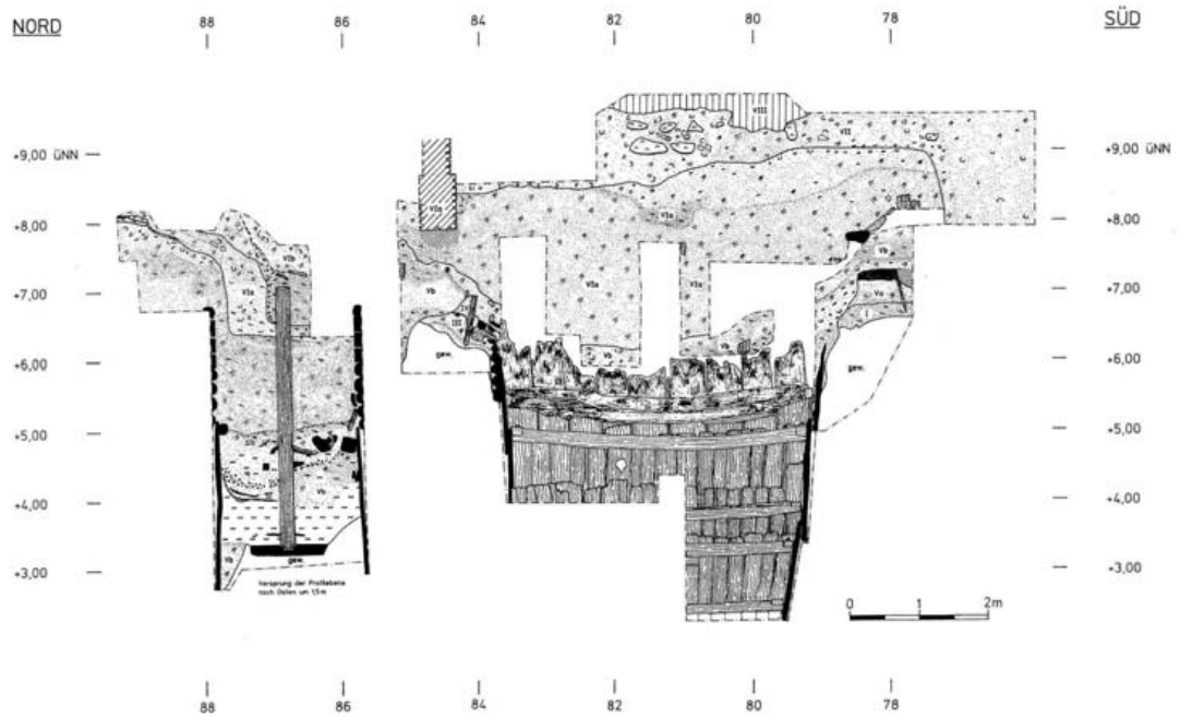
Abb. 120 Hansestadt Lübeck, Alfstraße-Fischstraße-Schüsselbuden. Ostprofil 10, Alfstraße 7/Fischstraße 8 (Achsen 76-89, Lage vgl. Abb. 11).
