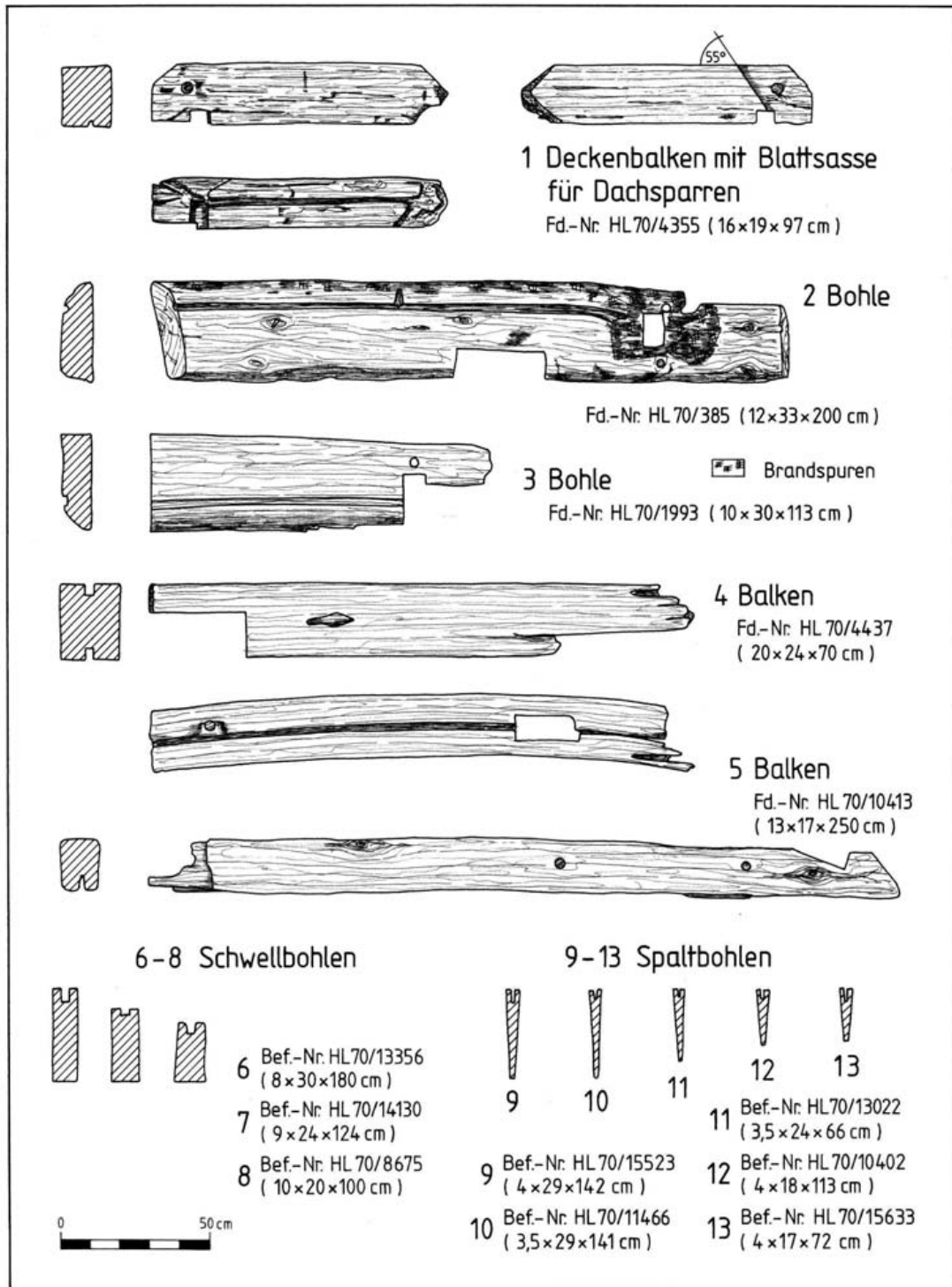
Abb. 94 Hansestadt Lübeck, Alfstraße-Fischstraße-Schüsselbuden. In verworfener Lage erfaßte Bauhölzer in Stabbauweise. 1 Deckenbalken mit Blattsasse (Alfstraße 9, Per. Vb). 2 Bohle (Fischstraße 12/14, Per. Vb). 3 Bohle (Fischstraße 12, Per. Vb). 4 Balken (Alfstraße 9, Periode Vb). 5 Balken (Fischstraße 8, Per. IV). 6 Schwellbohle (Fischstraße 8, Per. Vb). 7 Schwellbohle (Alfstraße 7, Per. Vb). 8 Schwellbohle (Alfstraße 9, Per. Vb). 9 Spaltbohle (Alfstraße 9, Peri. IV). 10 Spaltbohle (Fischstraße 10, Per. VIa). 11 Spaltbohle (Fischstraße 8, Per. VIa). 12 Spaltbohle (Alfstraße 11, Per. VIa). 13 Spaltbohle (Alfstraße 9, Per. VIa).
