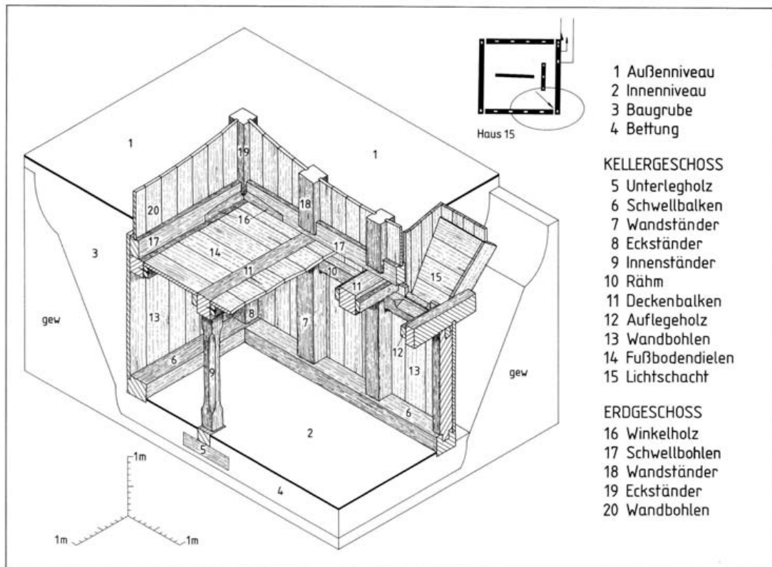
Abb. 96 Hansestadt Lübeck, Alfstraße-Fischstraße-Schüsselbuden. Isometrische Rekonstruktion zum Bauegefüge der unterkellerten Ständerbauten. Kellergeschoß Haus 15 (vgl. Abb. 57-63), Verbindung zum Erdgeschoß Haus 18 (vgl. Abb. 70-78).
