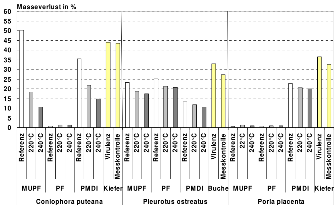
Abbildung 56: Masseverlust durch Coniophora puteana , Pleurotus ostreatus und Poria placenta nach 16wöchiger Inkubationszeit von OSB aus Kiefer. Die bei 220°C und 240°C vorbehandelten Strands sowie unbehandelte Referenzstrands wurden mit MUPF, PF und PMDI zu Platten verpresst.
