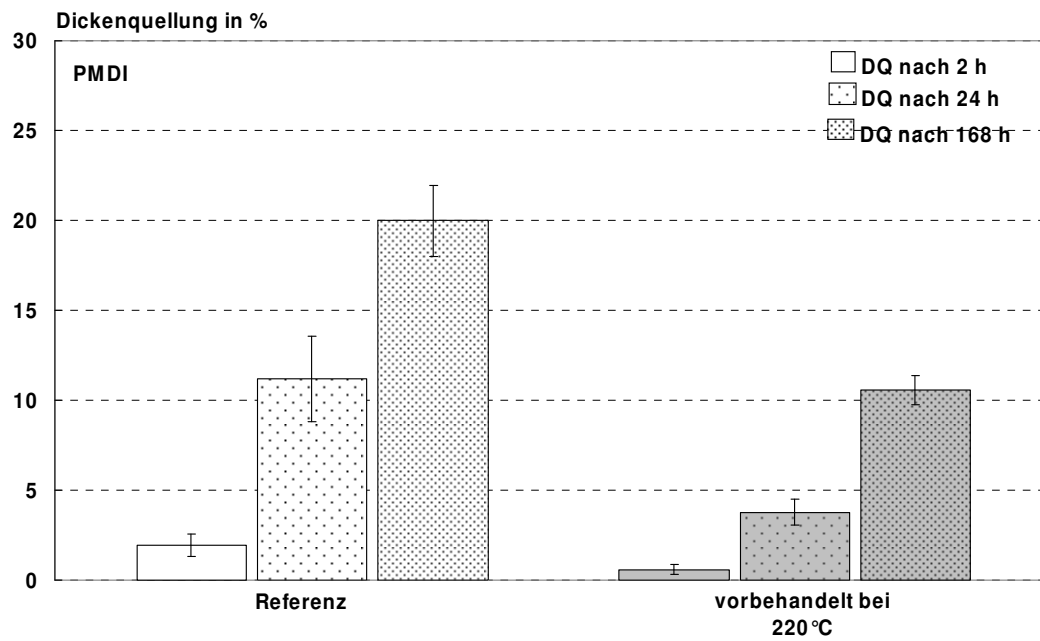
Abbildung 24: Dickenquellung (DQ) nach 2, 24 und 168 Stunden Wasserlagerung von OSB aus Pappel. Die bei 220°C vorbehandelten Strands sowie unbehandelte Referenzstrands wurden mit PMDI zu Platten verpresst.
