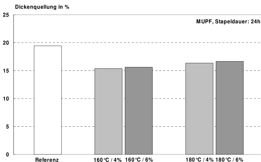
Abbildung 81: Irreversible Dickenquellung nach künstlicher Bewitterung und Klimatisierung bei 20°C und 65% r. Lf. von MUPF-gebundenen Platten, die bei 160°C bzw. 180°C für 24 Stunden im Stapel nachbehandelt wurden; die Feuchte der Platten war auf 4% bzw. 6% eingestellt.
