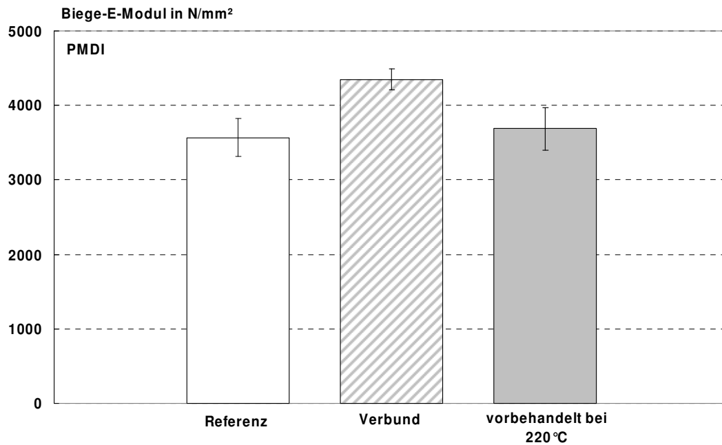
Abbildung 39: Biege-E-Modul PMDI-gebundener Fichtespanplatten aus unbehandelten und thermisch modifizierten Spänen sowie aus einem Verbund beider Spantypen.
