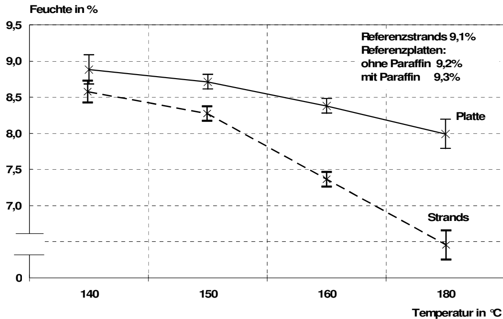
Abbildung 1: Gleichgewichtsfeuchte bei 20°C und 65% r. Lf. von OSB-Strands aus Kiefer, die bei 140°C bis 180°C in Luftatmosphäre vorbehandelt wurden, sowie daraus gefertigter Platten.
