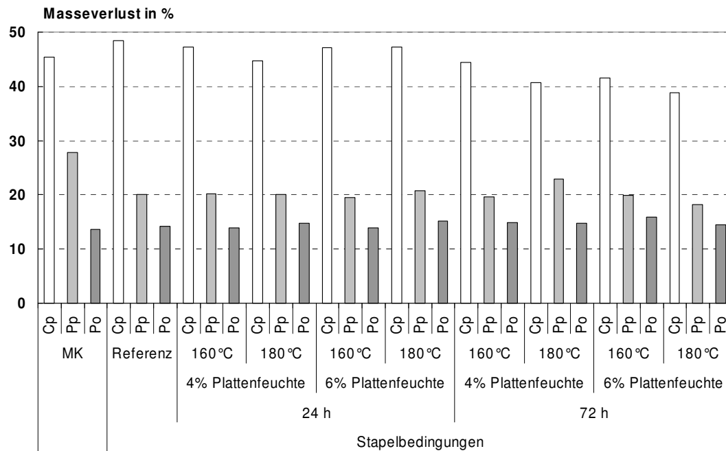
Abbildung 88: Masseverlust durch Coniophora puteana (Cp), Pleurotus ostreatus (Po) und Poria placenta (Pp) nach 16wöchiger Inkubationszeit von PMDI-gebundenen OSB aus Kiefer. Die Platten einer Feuchte von 4% bzw. 6% wurden durch Nachbehandlung im Stapel bei 160°C bzw. 180°C für 24 und 72 Stunden modifiziert.
