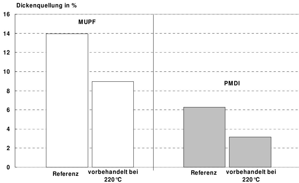
Abbildung 48: Irreversible Dickenquellung nach BAM-Zyklus von Spanplatten aus Fichte. Die bei 220°C vorbehandelten Späne sowie unbehandelte Referenzspäne wurden mit MUPF und PMDI zu Platten verpresst.
