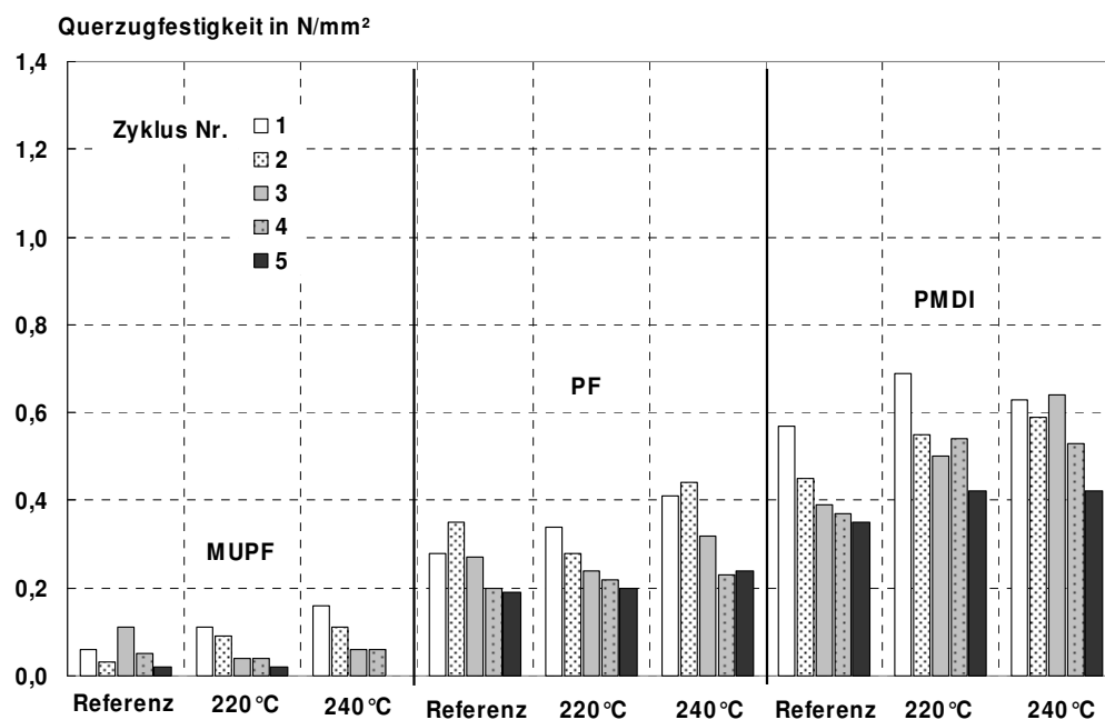
Abbildung 47: Querzugfestigkeit nach Zyklustest (2) von OSB aus Kiefer. Die bei 220°C und 240°C vorbehandelten Strands sowie unbehandelte Referenzstrands wurden mit MUPF, PF und PMDI zu Platten verpresst.
