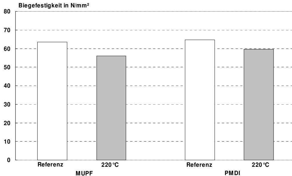
Abbildung 38: Biegefestigkeit MUPF- und PMDI-gebundener Fichtespanplatten aus unbehandelten und thermisch modifizierten Spänen, zusätzlich beschichtet mit Deckfurnieren aus Kiefer.
