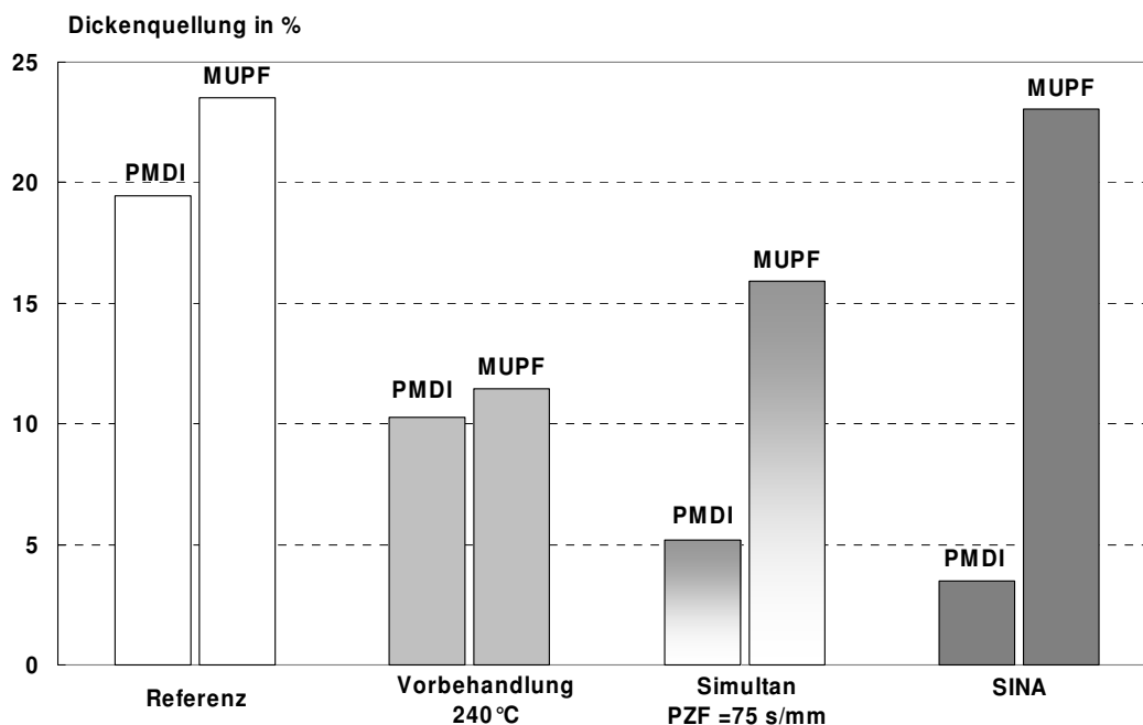
Abbildung 98: Dickenquellung nach 24 Stunden Wasserlagerung MUPF- und PMDI-gebundener OSB aus Kiefer, hergestellt nach verschiedenen Verfahren zur thermischen Modifizierung.
