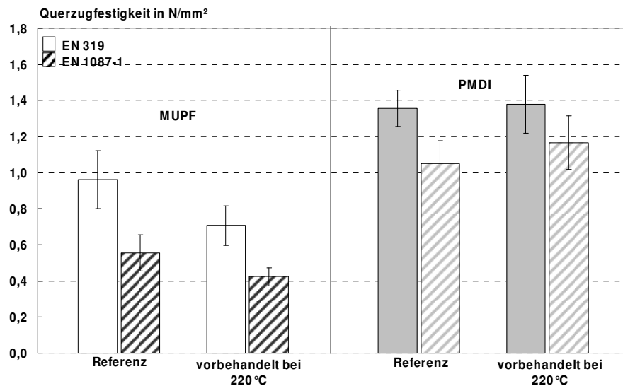
Abbildung 28: Querzugfestigkeit (QZ) trocken (EN 319) und nach Kochtest (EN 1087-1) von Spanplatten aus Fichte. Die bei 220°C vorbehandelten Späne sowie unbehandelte Referenzspäne wurden mit MUPF und PMDI zu Platten verpresst.
