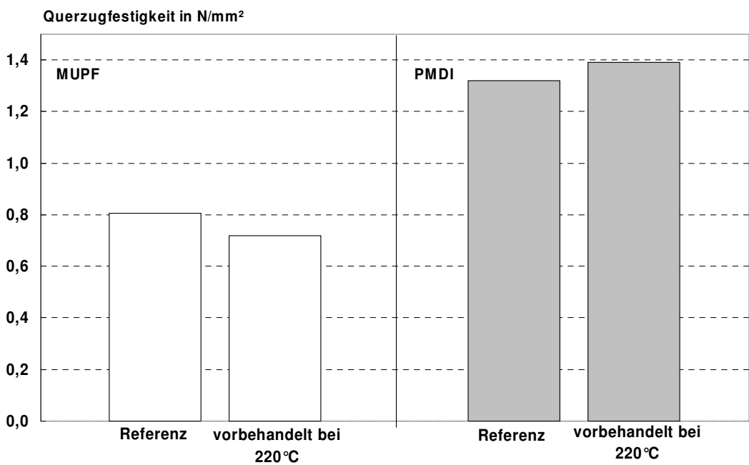
Abbildung 49: Querzugfestigkeit nach BAM-Zyklus von Spanplatten aus Fichte. Die bei 220°C vorbehandelten Späne sowie unbehandelte Referenzspäne wurden mit MUPF und PMDI zu Platten verpresst.
