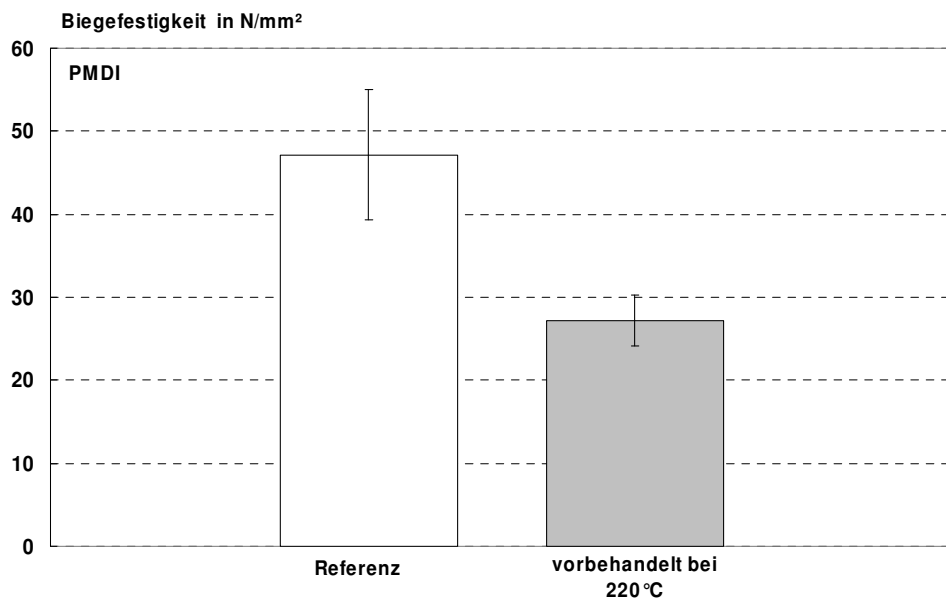
Abbildung 36: Biegefestigkeit von OSB aus Pappel. Die bei 220°C vorbehandelten Strands sowie unbehandelte Referenzstrands wurden mit PMDI zu Platten verpresst.
