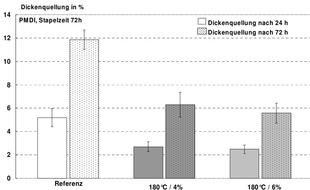
Abbildung 68: Dickenquellung nach 24 und 72 Stunden Wasserlagerung von PMDI-gebundenen Platten, die für 72 Stunden bei 180°C nachbehandelt wurden; die Feuchte der Platten war auf 4% bzw. 6% eingestellt.
