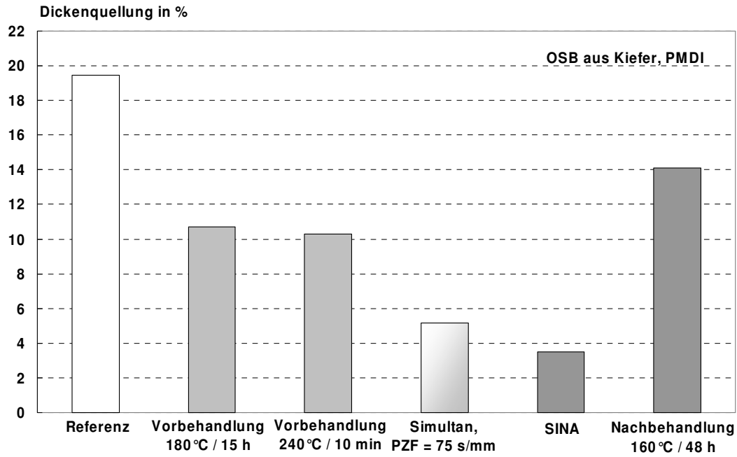
Abbildung 96: Dickenquellung nach 24 Stunden Wasserlagerung PMDI-gebundener OSB aus Kiefer, hergestellt nach verschiedenen Verfahren zur thermischen Modifizierung.
