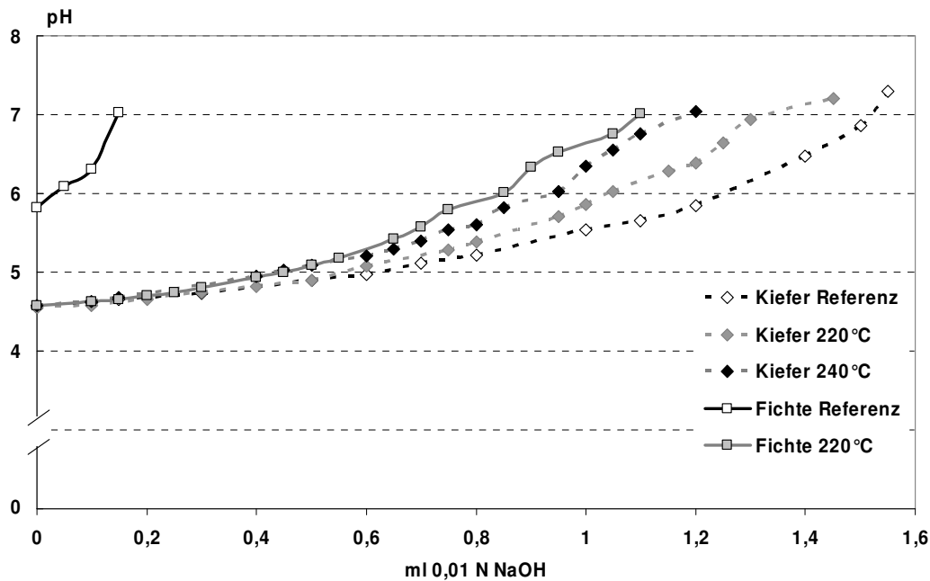
Abbildung 14: Titrationskurven zur Bestimmung der Pufferkapazität von Strands aus Kiefer und Fichtespänen nach Vorbehandlung bei 220°C bzw. 240°C im Vergleich zur unbehandelten Referenz.
