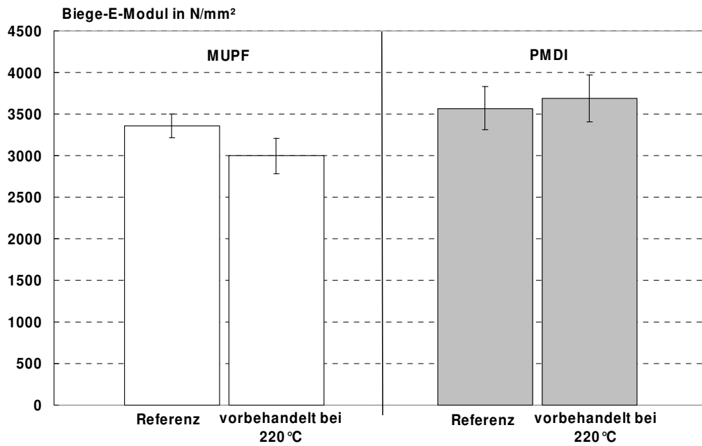
Abbildung 33: Biege-Elastizitätsmodul von Spanplatten aus Fichte. Die bei 220°C vorbehandelten Späne sowie unbehandelte Referenzspäne wurden mit MUPF und PMDI zu Platten verpresst.
