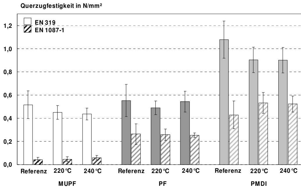
Abbildung 27: Querzugfestigkeit (QZ) trocken (EN 319) und nach Kochtest (EN 1087-1) von OSB aus Kiefer. Die bei 220°C und 240°C vorbehandelten Strands sowie unbehandelte Referenzstrands wurden mit MUPF, PF und PMDI zu Platten verpresst.
