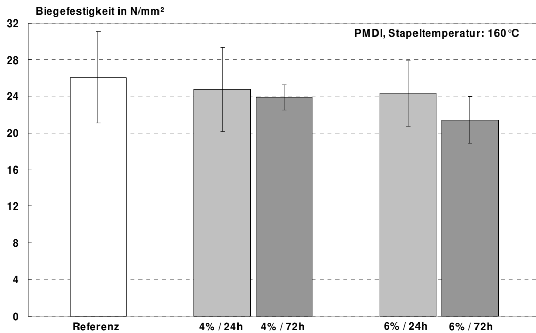
Abbildung 79: Biegefestigkeit von PMDI-gebundenen Platten, die bei 160°C für 24 bzw. 72 Stunden im Stapel nachbehandelt wurden; die Feuchte der Platten war auf 4% bzw. 6% eingestellt.
