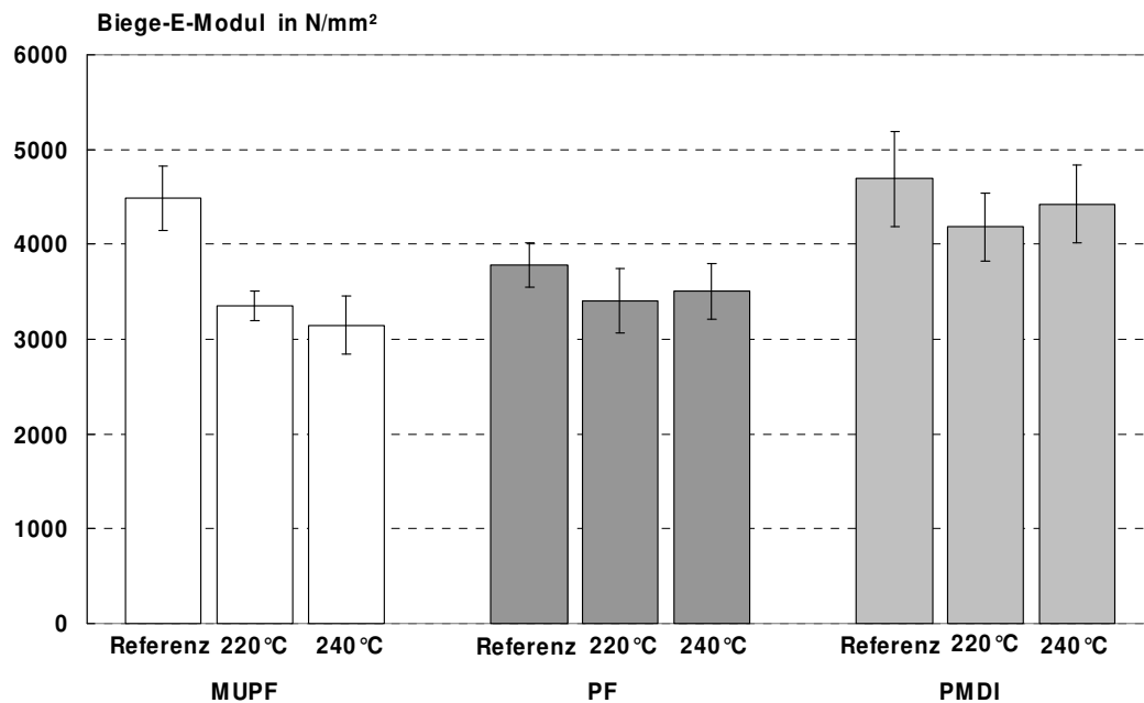
Abbildung 31: Biege-Elastizitätsmodul von OSB aus Kiefer. Die bei 220°C und 240°C vorbehandelten Strands sowie unbehandelte Referenzstrands wurden mit MUPF, PF und PMDI zu Platten verpresst.
