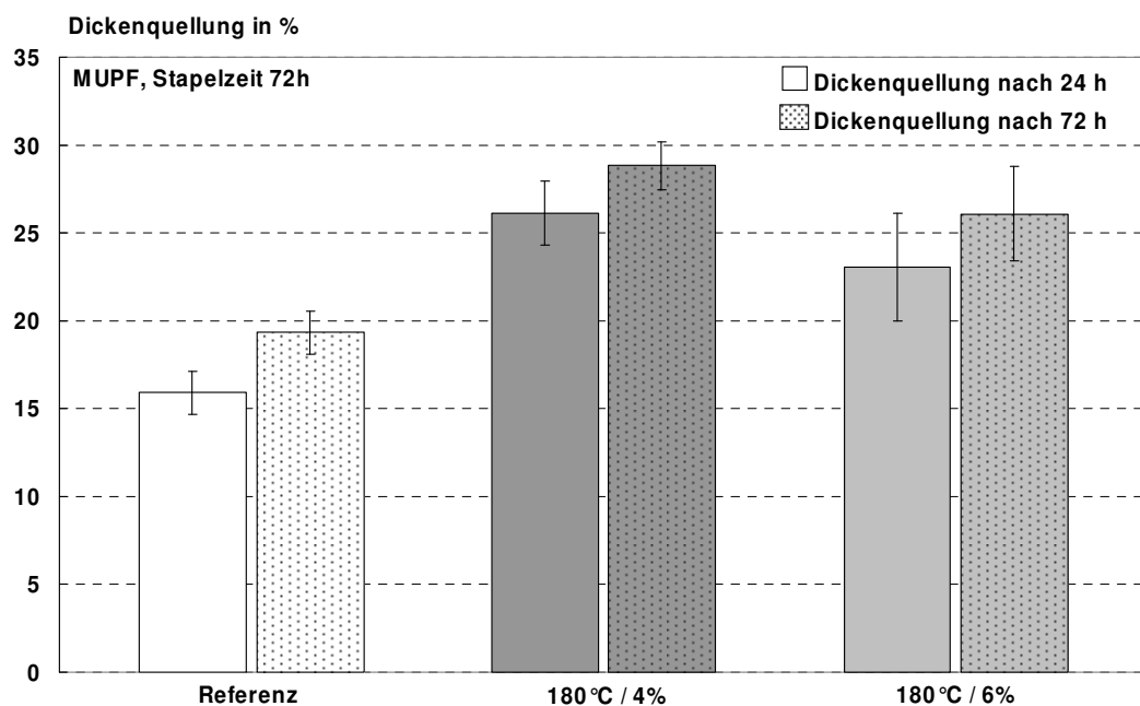
Abbildung 64: Dickenquellung nach 24 und 72 Stunden Wasserlagerung von MUPF-gebundenen Platten, die für 72 Stunden bei 180°C nachbehandelt wurden; die Feuchte der Platten war auf 4% bzw. 6% eingestellt.
