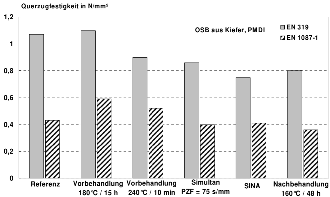
Abbildung 97: Querzugfestigkeit nach EN 319 und EN 1087-1 PMDI-gebundener OSB aus Kiefer, hergestellt nach verschiedenen Verfahren zur thermischen Modifizierung.
