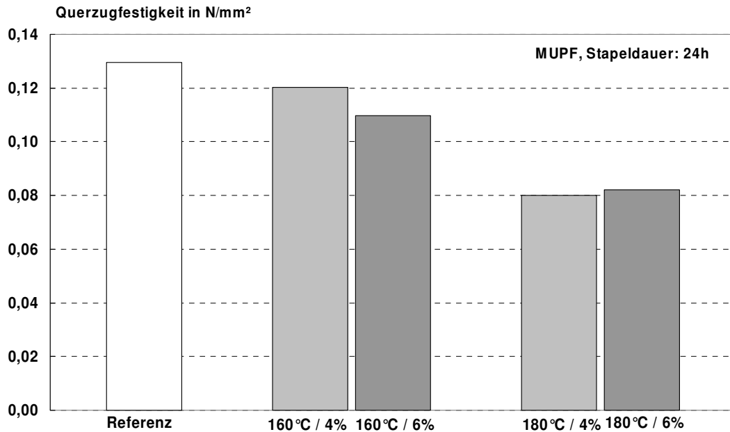
Abbildung 82: Querzugfestigkeit nach künstlicher Bewitterung von MUPF-gebundenen Platten, die bei 160°C bzw. 180°C für 24 Stunden im Stapel nachbehandelt wurden; die Feuchte der Platten war auf 4% bzw. 6% eingestellt.
