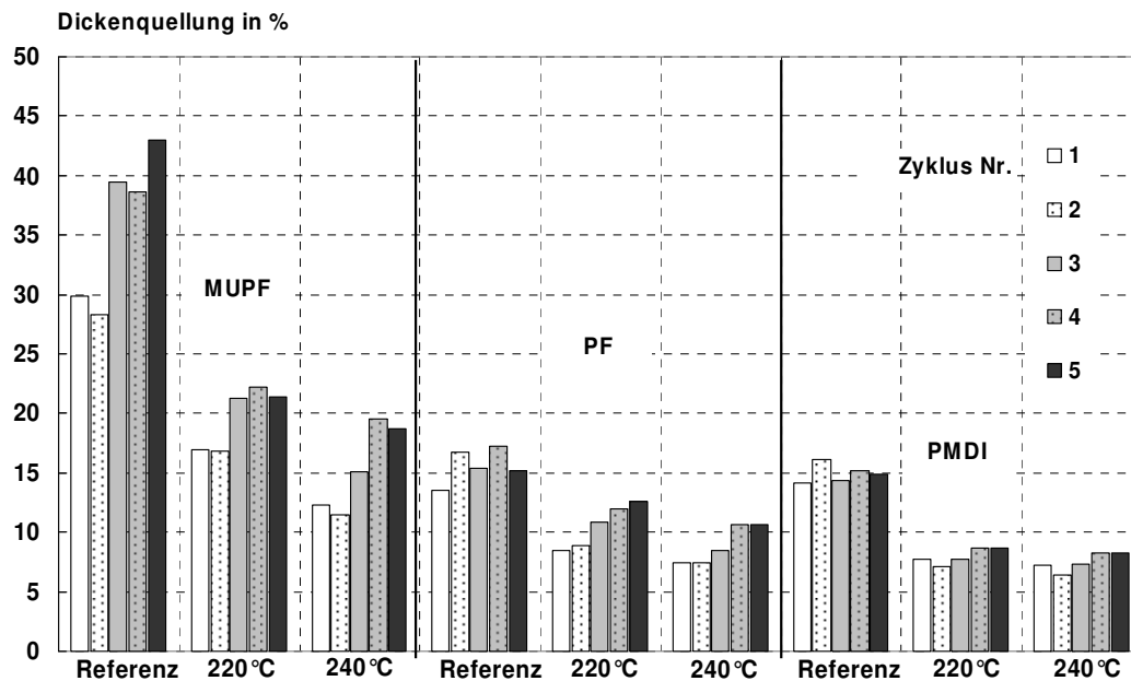
Abbildung 46: Irreversible Dickenquellung nach Zyklustest (2) von OSB aus Kiefer. Die bei 220°C und 240°C vorbehandelten Strands sowie unbehandelte Referenzstrands wurden mit MUPF, PF und PMDI zu Platten verpresst.
