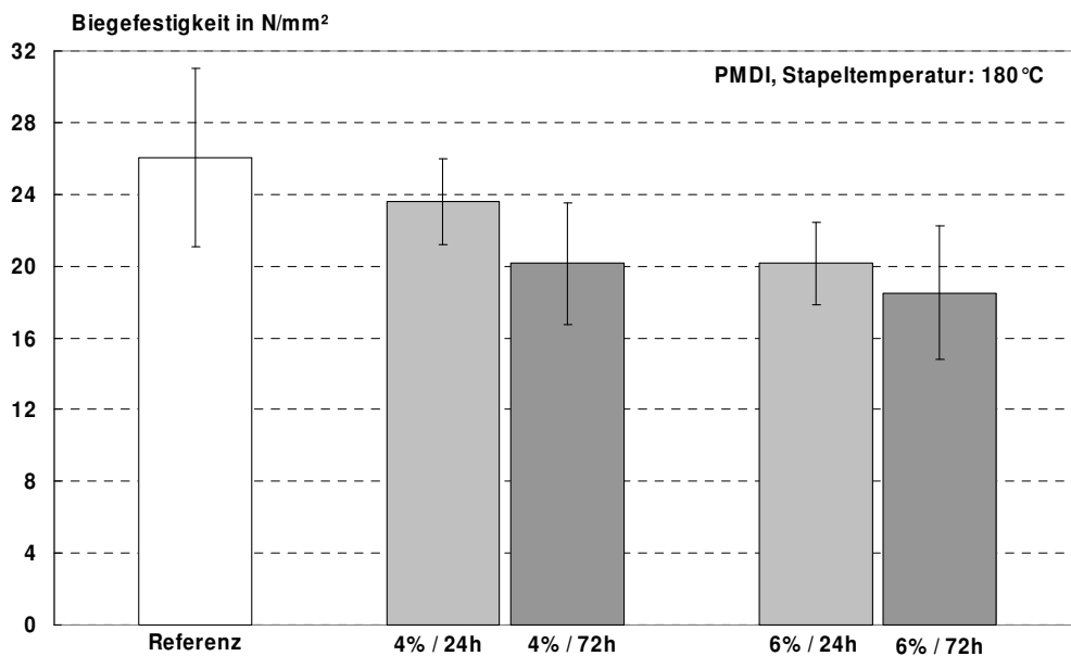
Abbildung 80: Biegefestigkeit von PMDI-gebundenen Platten, die bei 180°C für 24 bzw. 72 Stunden im Stapel nachbehandelt wurden; die Feuchte der Platten war auf 4% bzw. 6% eingestellt.
