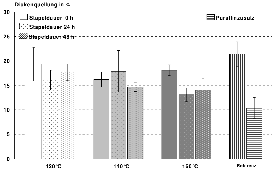
Abbildung 90: Dickenquellung nach 24 Stunden Wasserlagerung von OSB, die bei 120°C, 140°C bzw. 160°C für 24 bzw. 48 Stunden im Stapel nachbehandelt wurden im Vergleich zur Referenz. Die Presszeit hing von der angestrebten Stapeltemperatur ab (Stapeldauer 0 h).
