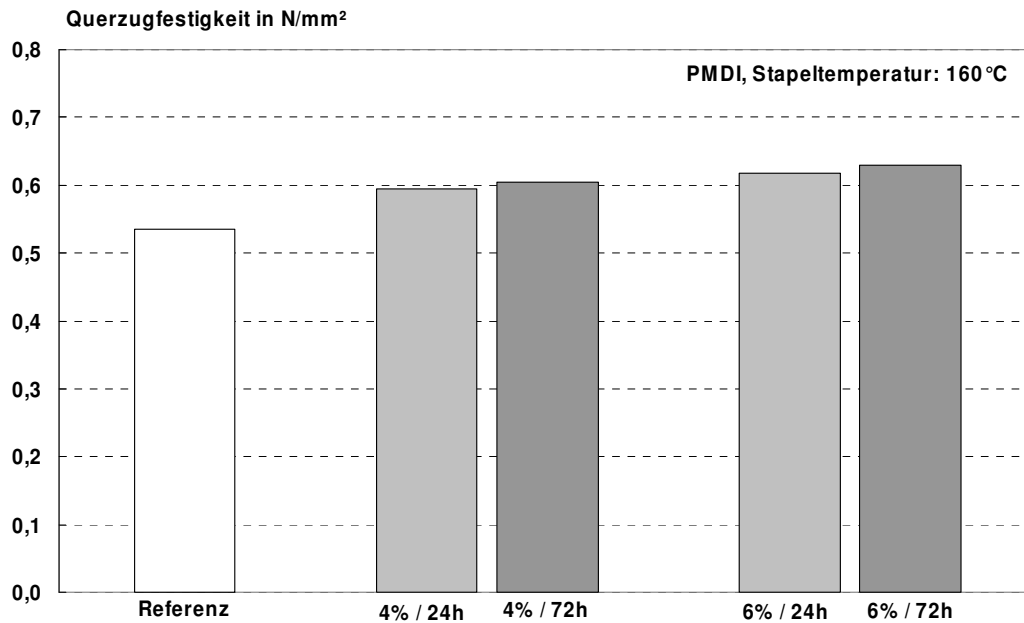
Abbildung 85: Querzugfestigkeit nach künstlicher Bewitterung von PMDI-gebundenen Platten, die bei 160°C für 24 bzw. 72 Stunden im Stapel nachbehandelt wurden; die Feuchte der Platten war auf 4% bzw. 6% eingestellt.
