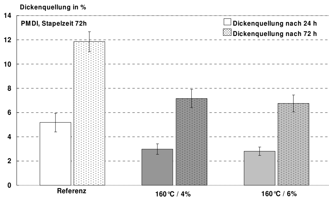
Abbildung 67: Dickenquellung nach 24 und 72 Stunden Wasserlagerung von PMDI-gebundenen Platten, die für 72 Stunden bei 160°C nachbehandelt wurden; die Feuchte der Platten war auf 4% bzw. 6% eingestellt.
