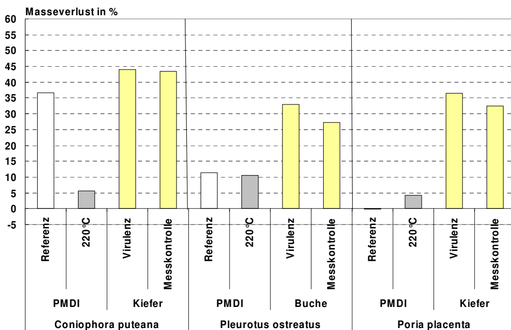
Abbildung 58: Masseverlust durch Coniophora puteana , Pleurotus ostreatus und Poria placenta nach 16wöchiger Inkubationszeit von OSB aus Pappel. Die bei 220°C vorbehandelten Strands sowie unbehandelte Referenzstrands wurden mit PMDI zu Platten verpresst.
