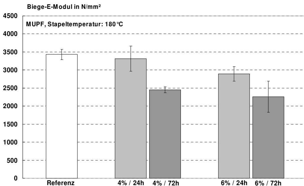
Abbildung 74: Biege-E-Modul von MUPF-gebundenen Platten, die bei 180°C für 24 bzw. 72 Stunden im Stapel nachbehandelt wurden; die Feuchte der Platten war auf 4% bzw. 6% eingestellt.
