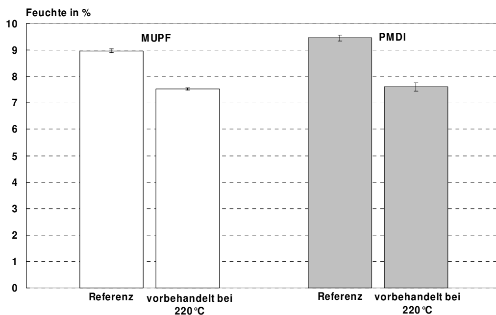
Abbildung 19: Gleichgewichtsfeuchte bei 20°C und 65% r. Lf. von Spanplatten aus Fichte. Die bei 220°C vorbehandelten Späne sowie unbehandelte Referenzspäne wurden mit MUPF und PMDI zu Platten verpresst.
