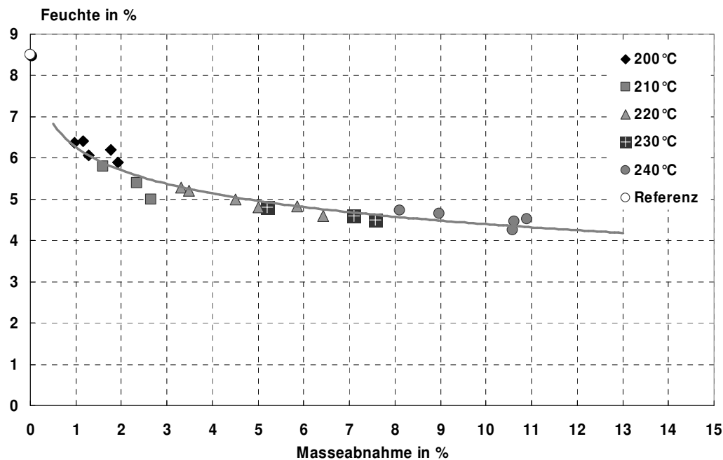
Abbildung 13: Gleichgewichtsfeuchte bei 20°C / 65% von Pappel-Strands in Abhängigkeit der Masseabnahme durch thermische Modifizierung gemäß Abbildung 12.
