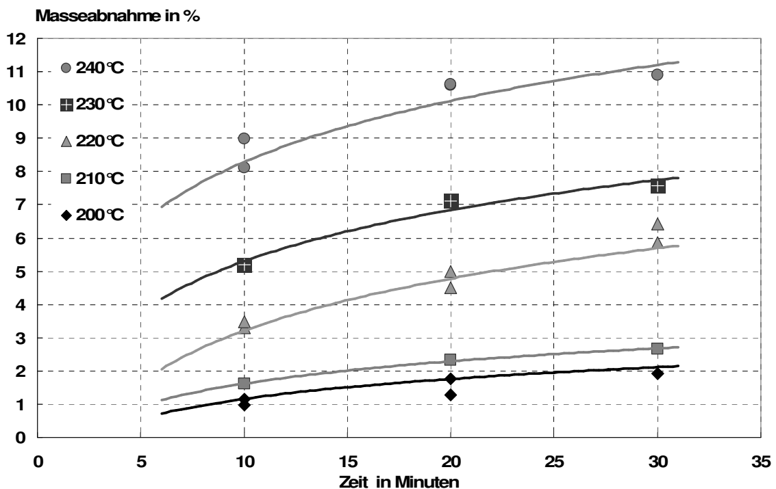
Abbildung 12: Masseabnahme von Pappel-Strands durch thermische Modifizierung bei 200°C bis 240°C in Abhängigkeit der Behandlungsdauer.
