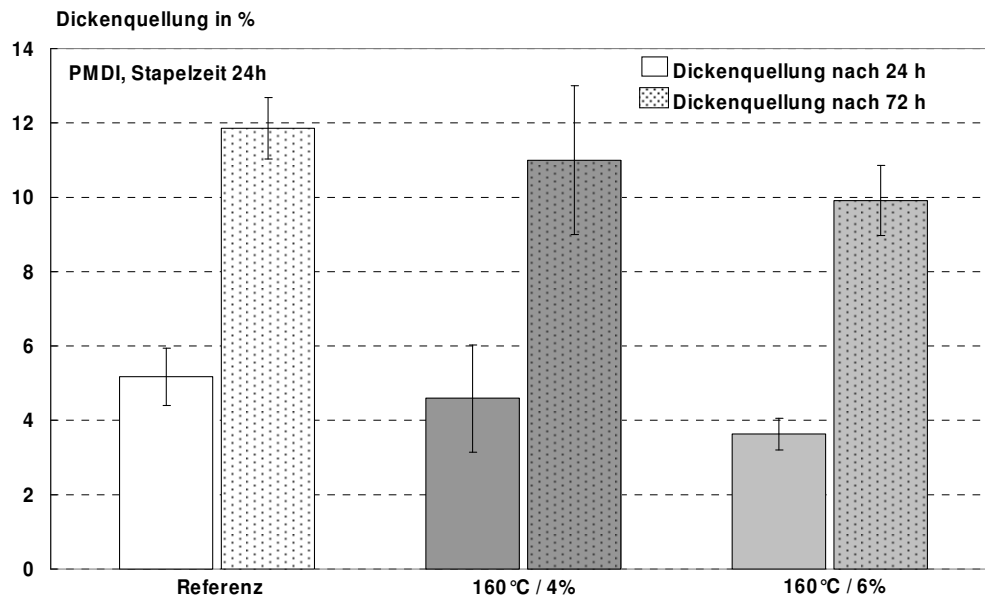
Abbildung 65: Dickenquellung nach 24 und 72 Stunden Wasserlagerung von PMDI-gebundenen Platten, die für 24 Stunden bei 160°C nachbehandelt wurden; die Feuchte der Platten war auf 4% bzw. 6% eingestellt.
