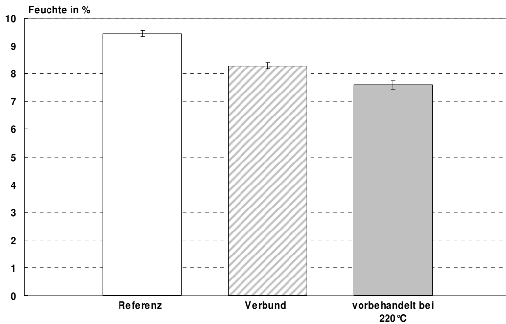
Abbildung 42: Feuchtaufnahme bei 20°C und 65% r. Lf. PMDI-gebundener Fichtespanplatten aus unbehandelten und thermisch modifizierten Spänen sowie einem Verbund aus beiden Spantypen.
