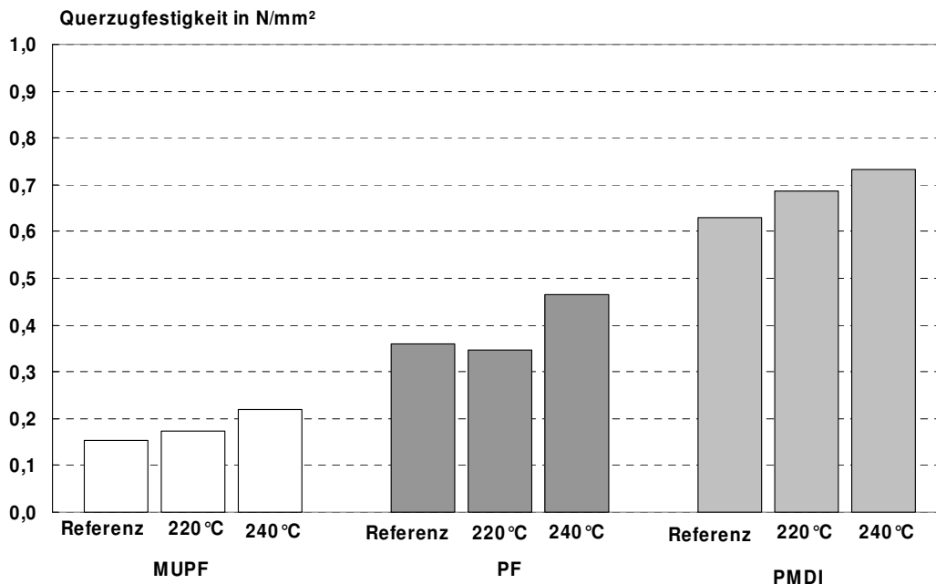
Abbildung 45: Querkzugfestigkeit nach BAM-Zyklus von OSB aus Kiefer. Die bei 220^\circ\text{C} und 240^\circ\text{C} vorbehandelten Strands sowie unbehandelte Referenzstrands wurden mit MUPF, PF und PMDI zu Platten verpresst.
