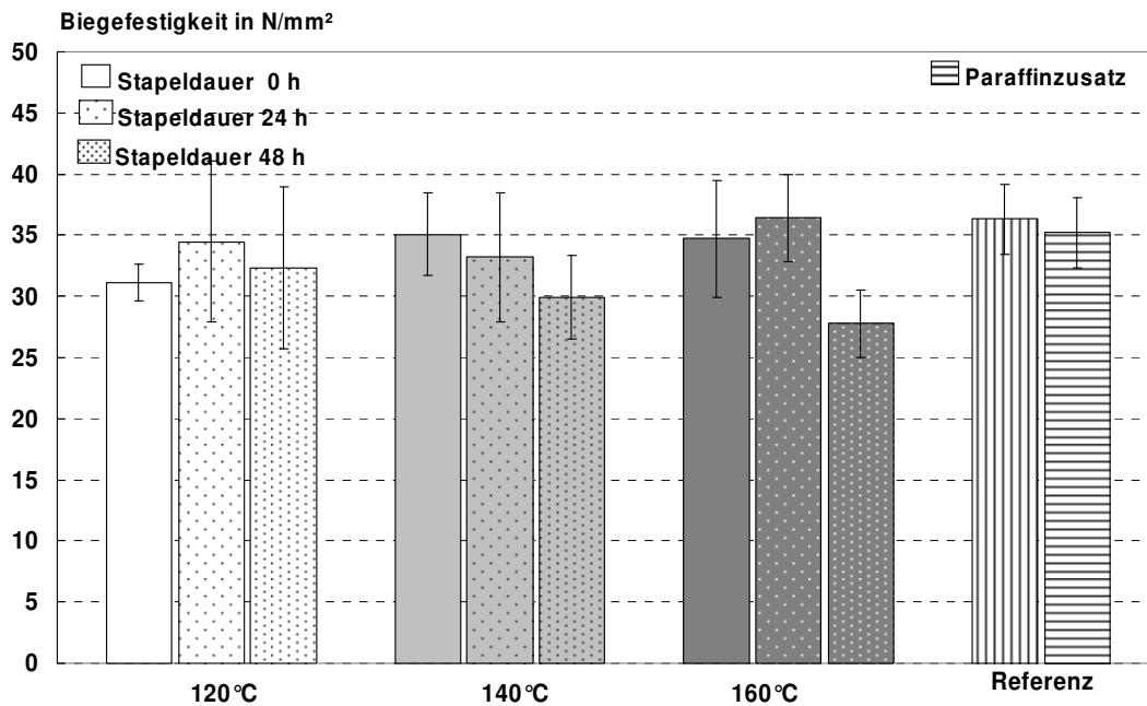
Abbildung 94: Biegefestigkeit von OSB, die bei 120°C, 140°C bzw. 160°C für 24 bzw. 48 Stunden im Stapel nachbehandelt wurden im Vergleich zur Referenz. Die Presszeit hing von der angestrebten Stapeltemperatur ab (Stapeldauer 0 h).
