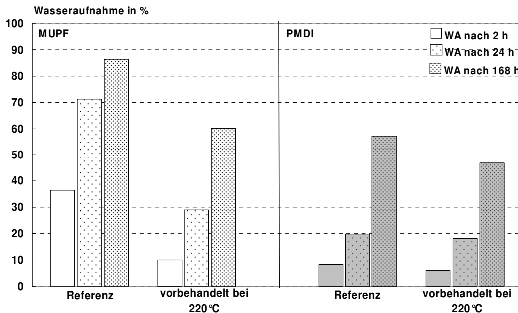
Abbildung 21: Wasseraufnahme (WA) nach 2, 24 und 168 Stunden Wasserlagerung von Spanplatten aus Fichte. Die bei 220°C vorbehandelten Späne sowie unbehandelte Referenzspäne wurden mit MUPF und PMDI zu Platten verpresst.
