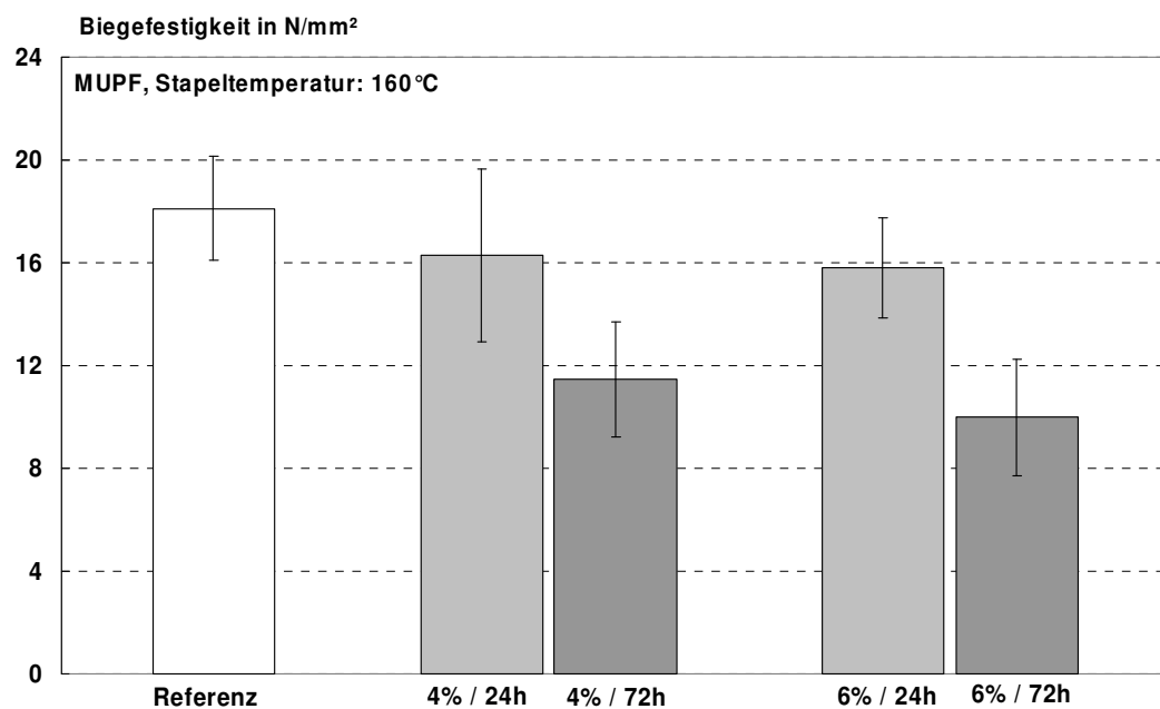
Abbildung 75: Biegefestigkeit von MUPF-gebundenen Platten, die bei 160°C für 24 bzw. 72 Stunden im Stapel nachbehandelt wurden; die Feuchte der Platten war auf 4% bzw. 6% eingestellt.
