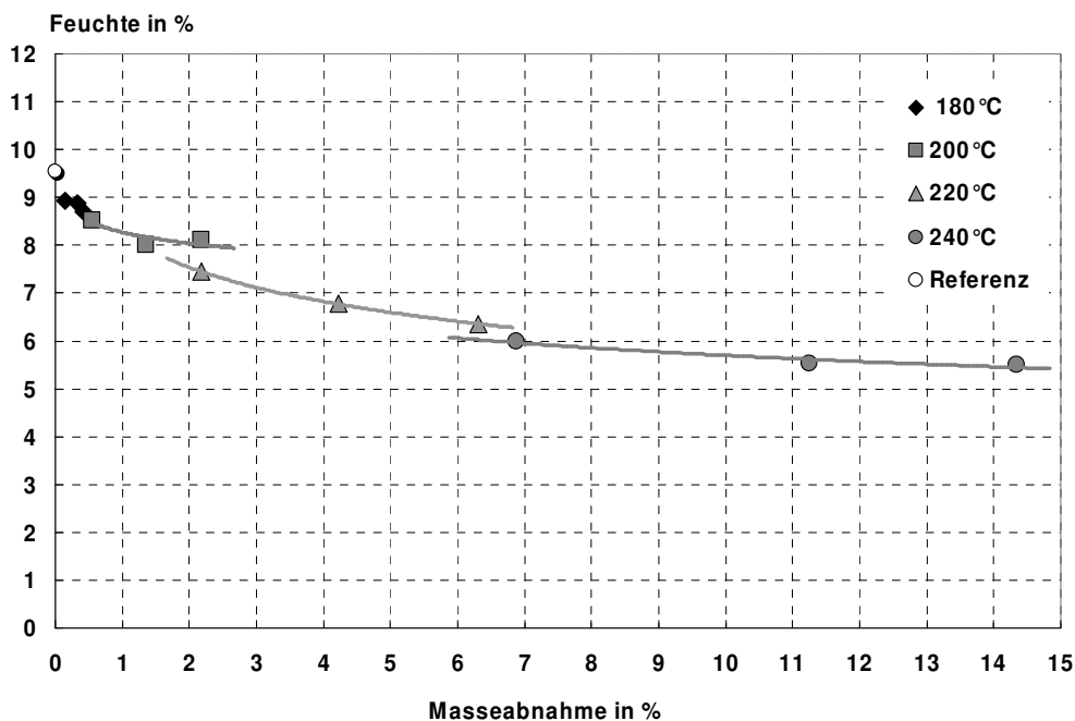
Abbildung 9: Gleichgewichtsfeuchte bei 20°C und 65% r. Lf. von Kiefer-Strands in Abhängigkeit der Masseabnahme infolge thermischer Modifizierung gemäß Abbildung 8.
