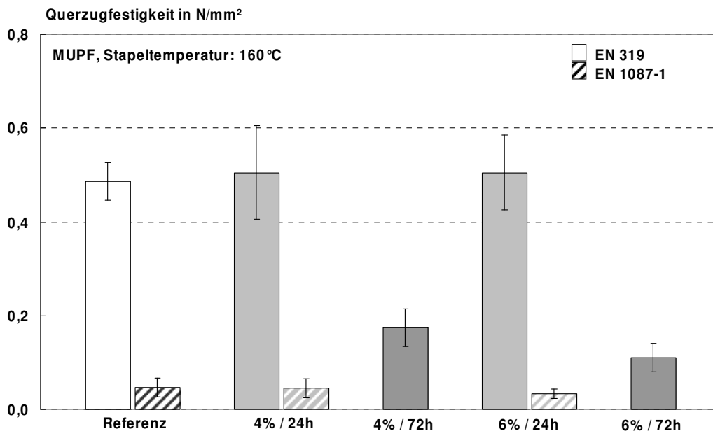
Abbildung 69: Querkzugfestigkeit trocken (EN 319) sowie nach Kochtest (EN 1087-1) von MUPF-gebundenen Platten, die bei 160°C für 24 bzw. 72 Stunden im Stapel nachbehandelt wurden; die Feuchte der Platten war auf 4% bzw. 6% eingestellt.
