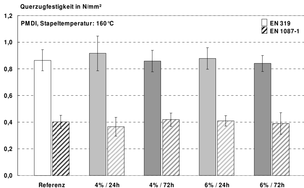
Abbildung 71: Querzugfestigkeit trocken (EN 319) sowie nach Kochtest (EN 1087-1) von PMDI-gebundenen Platten, die bei 160°C für 24 bzw. 72 Stunden im Stapel nachbehandelt wurden; die Feuchte der Platten war auf 4% bzw. 6% eingestellt.
