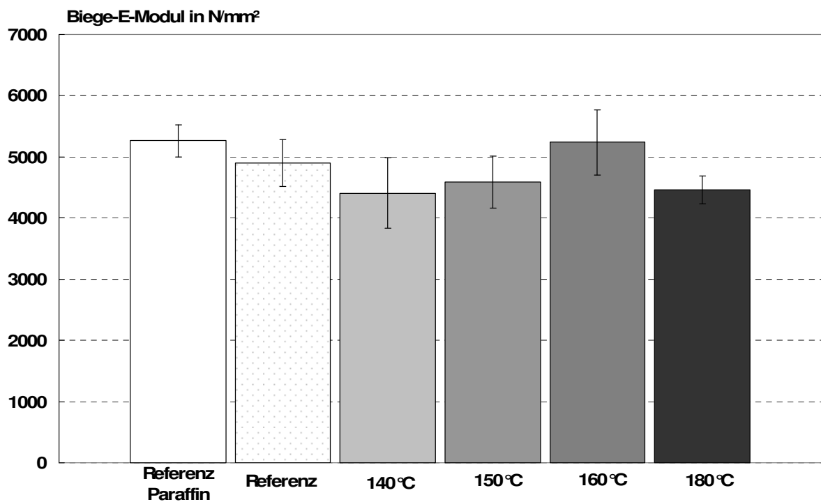
Abbildung 5: Biege-E-Modul PMDI-gebundener Kiefer-OSB, deren Strands bei 140°C bis 180°C thermisch modifiziert wurden.
