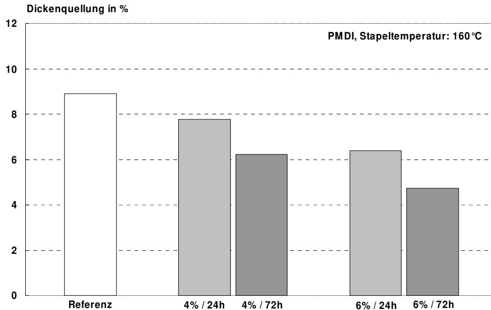
Abbildung 83: Irreversible Dickenquellung nach künstlicher Bewitterung und Klimatisierung bei 20°C und 65% r. Lf. von PMDI-gebundenen Platten, die bei 160°C für 24 bzw. 72 Stunden im Stapel nachbehandelt wurden; die Feuchte der Platten war auf 4% bzw. 6% eingestellt.
