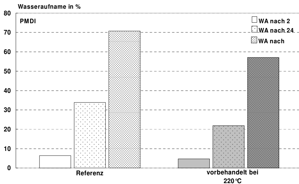
Abbildung 25: Wasseraufnahme (WA) nach 2, 24 und 168 Stunden Wasserlagerung von OSB aus Pappel. Die bei 220°C vorbehandelten Strands sowie unbehandelte Referenzstrands wurden mit PMDI zu Platten verpresst.
