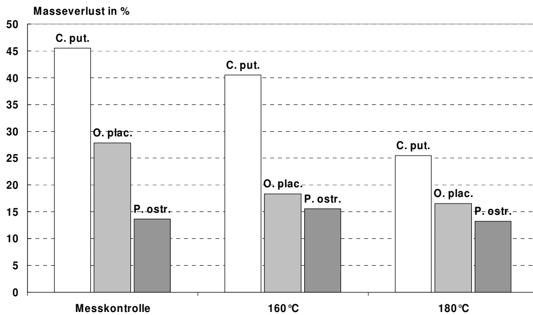
Abbildung 6: Dauerhaftigkeit gegen Pilzabbau PMDI-gebundener Kiefer-OSB, deren Strands bei 160°C und 180°C thermisch modifiziert wurden.
