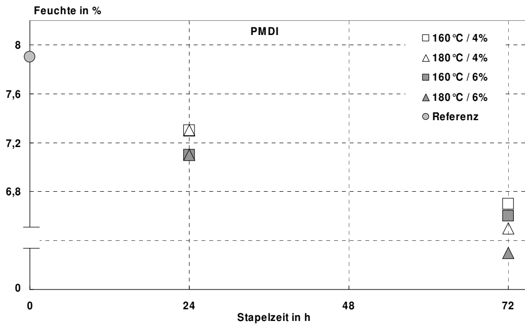
Abbildung 60: Gleichgewichtsfeuchte bei 20°C und 65% r. Lf. PMDI-gebundener OSB infolge Nachbehandlung im Stapel im Vergleich zur Referenz.
