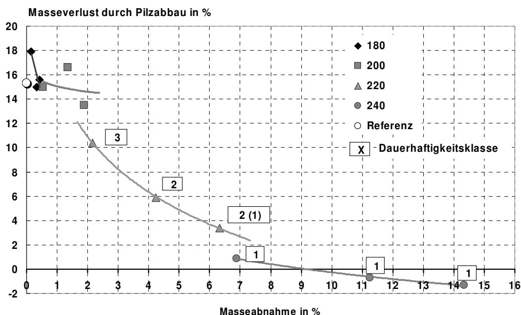
Abbildung 10: Masseverlust von Kiefern-Strands durch Pilzabbau ( Poria placenta ) in Abhängigkeit der Masseabnahme durch thermische Modifizierung gemäß Abbildung 8.
