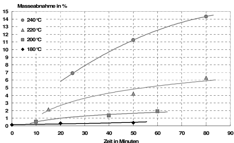
Abbildung 8: Masseabnahme von Kiefern-Strands durch thermische Modifizierung bei Temperaturen von 180°C bis 240°C in Abhängigkeit der Behandlungsdauer.
