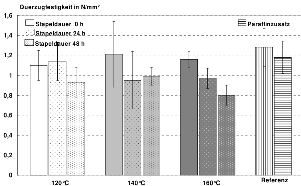
Abbildung 91: Querzugfestigkeit nach EN 319 von OSB, die bei 120°C, 140°C bzw. 160°C für 24 bzw. 48 Stunden im Stapel nachbehandelt wurden im Vergleich zur Referenz.
