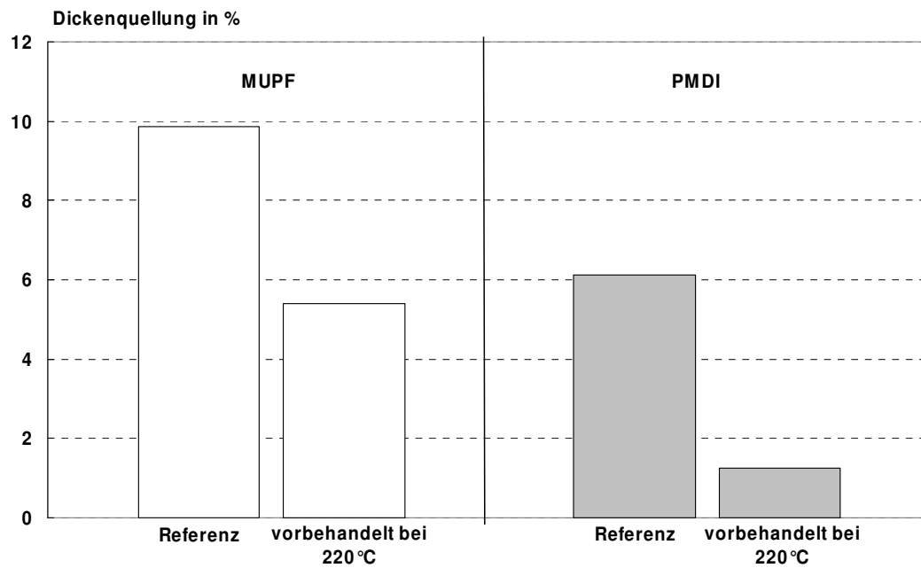
Abbildung 22: Irreversible Dickenquellung (IDQ) nach 168 Stunden Wasserlagerung von Spanplatten aus Fichte. Die bei 220°C vorbehandelten Späne sowie unbehandelte Referenzspäne wurden mit MUPF und PMDI zu Platten verpresst.
