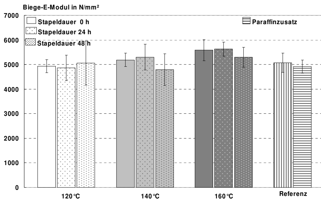
Abbildung 93: Biege-E-Modul von OSB, die bei 120°C, 140°C bzw. 160°C für 24 bzw. 48 Stunden im Stapel nachbehandelt wurden im Vergleich zur Referenz. Die Presszeit hing von der angestrebten Stapeltemperatur ab (Stapeldauer 0 h).
