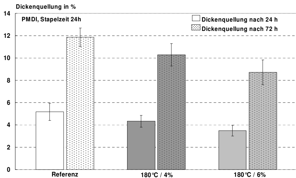
Abbildung 66: Dickenquellung nach 24 und 72 Stunden Wasserlagerung von PMDI-gebundenen Platten, die für 24 Stunden bei 180°C nachbehandelt wurden; die Feuchte der Platten war auf 4% bzw. 6% eingestellt.
