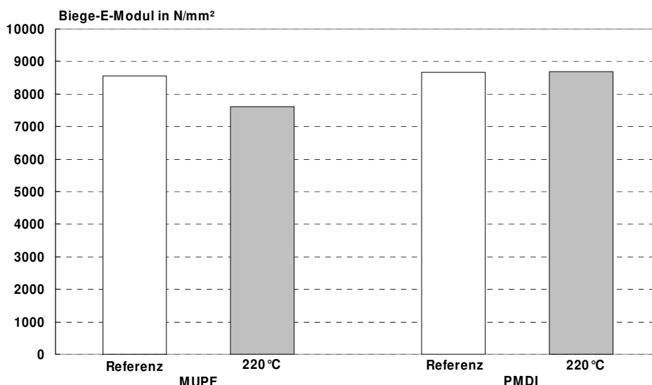
Abbildung 37: Biege-E-Modul MUPF- und PMDI-gebundener Fichtespanplatten aus unbehandelten und thermisch modifizierten Spänen, die zusätzlich mit Deckfurnieren aus Kiefer beschichtet wurden.
