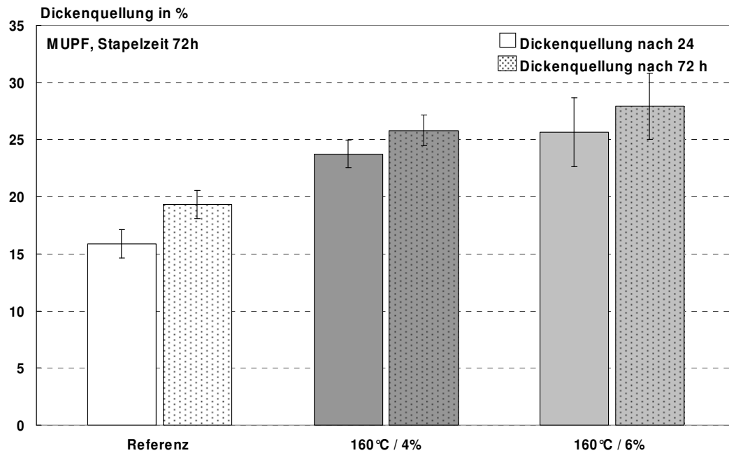
Abbildung 63: Dickenquellung nach 24 und 72 Stunden Wasserlagerung von MUPF-gebundenen Platten, die für 72 Stunden bei 160°C nachbehandelt wurden; die Feuchte der Platten war auf 4% bzw. 6% eingestellt.
