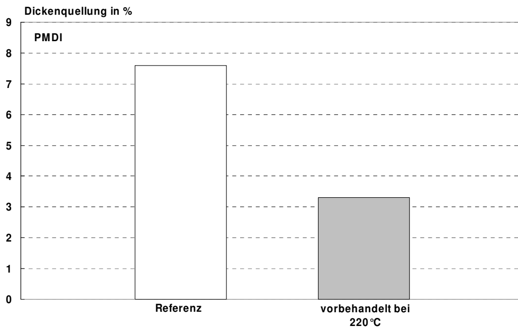
Abbildung 26: Irreversible Dickenquellung (IDQ) nach 168 Stunden Wasserlagerung von OSB aus Pappel. Die bei 220°C vorbehandelten Strands sowie unbehandelte Referenzstrands wurden mit PMDI zu Platten verpresst.
