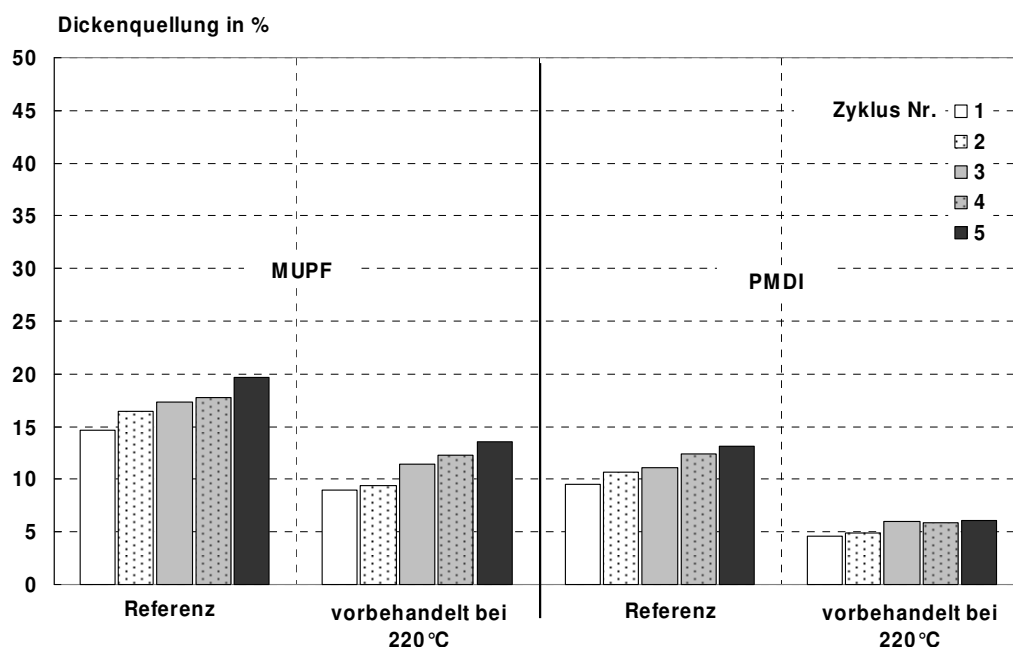
Abbildung 50: Irreversible Dickenquellung nach Zyklustest (2) von Spanplatten aus Fichte. Die bei 220°C vorbehandelten Späne sowie unbehandelte Referenzspäne wurden mit MUPF und PMDI zu Platten verpresst.
