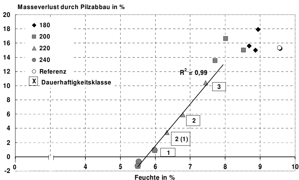
Abbildung 11: Masseverlust von Kiefern-Strands durch Pilzabbau ( Poria placenta ) in Abhängigkeit der Gleichgewichtsfeuchte bei 20°C / 65% gemäß Abbildung 9.
