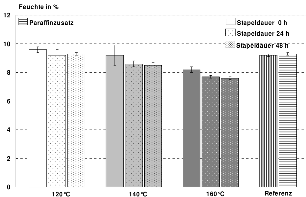
Abbildung 89: Gleichgewichtsfeuchte bei 20°C und 65% r. Lf. von OSB, die bei 120°C, 140°C bzw. 160°C für 24 bzw. 48 Stunden im Stapel nachbehandelt wurden im Vergleich zur Referenz. Die Presszeit hing von der angestrebten Stapeltemperatur ab (Stapeldauer 0 h).
