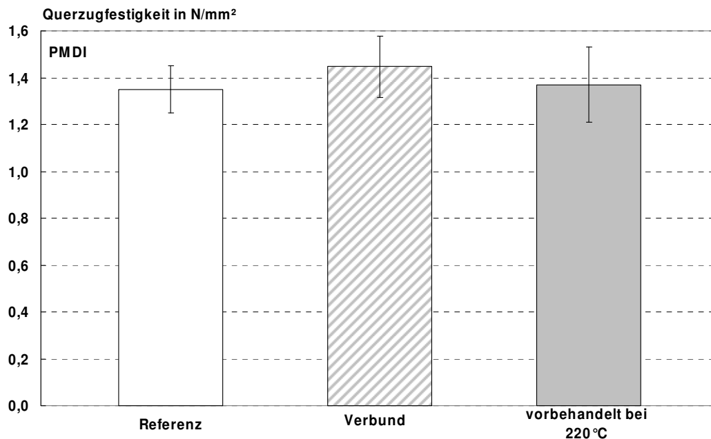
Abbildung 41: Querzugfestigkeit PMDI-gebundener Fichtespanplatten aus unbehandelten und thermisch modifizierten Spänen sowie aus einem Verbund beider Spantypen.
