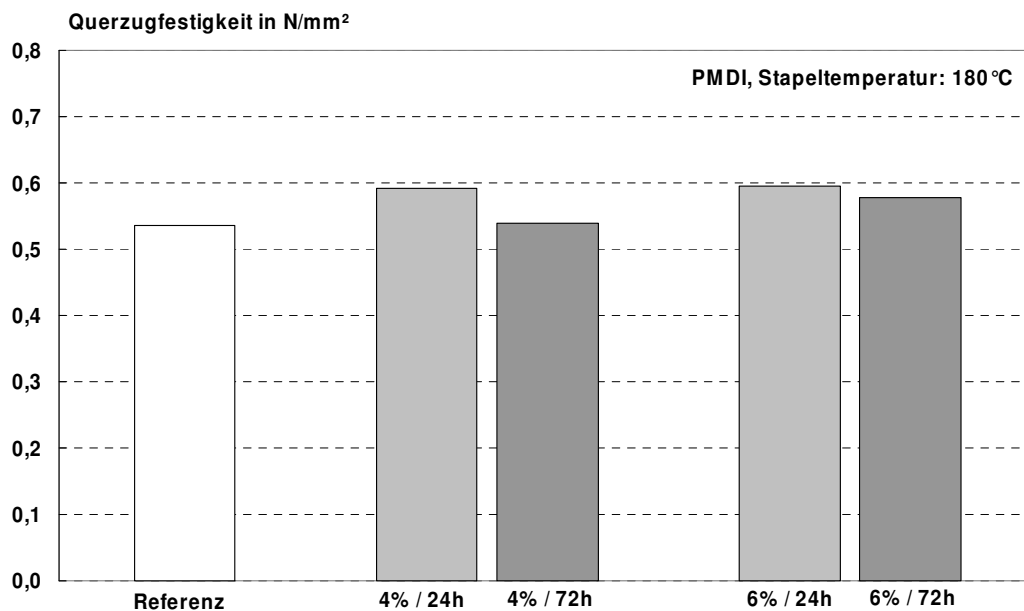
Abbildung 86: Querzugfestigkeit nach künstlicher Bewitterung von PMDI-gebundenen Platten, die bei 180°C für 24 bzw. 72 Stunden im Stapel nachbehandelt wurden; die Feuchte der Platten war auf 4% bzw. 6% eingestellt.
