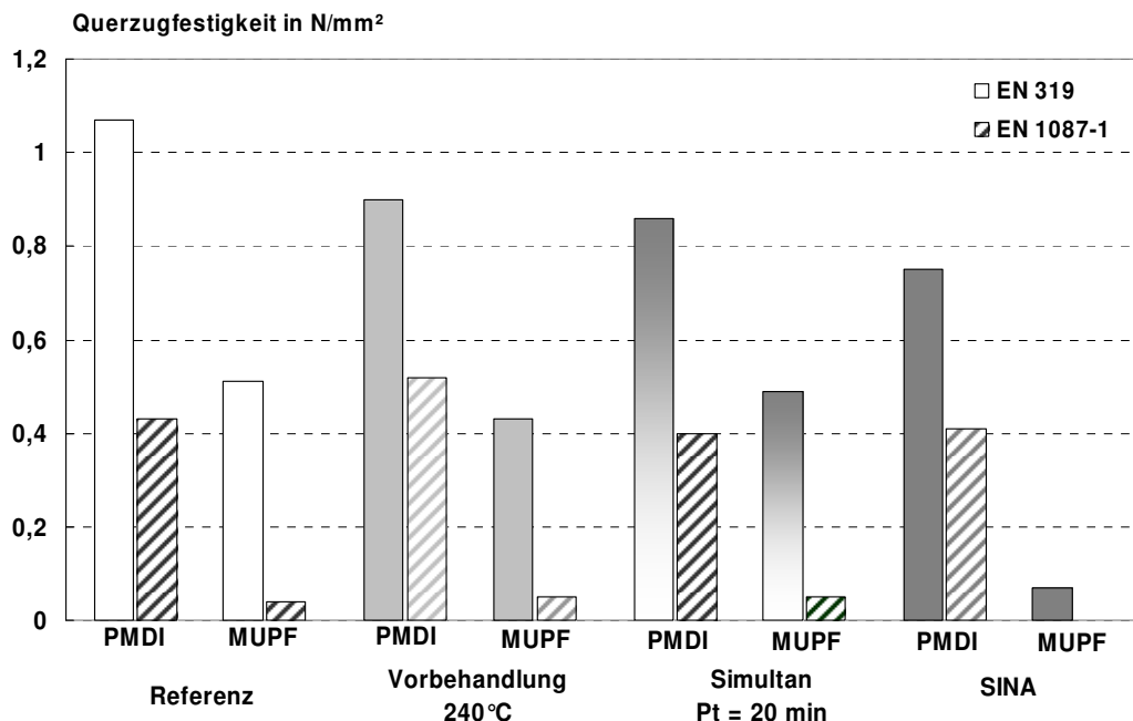
Abbildung 99: Querkzugfestigkeit nach EN 319 und EN 1087-1 MUPF- und PMDI-gebundener OSB aus Kiefer, hergestellt nach verschiedenen Verfahren zur thermischen Modifizierung.
