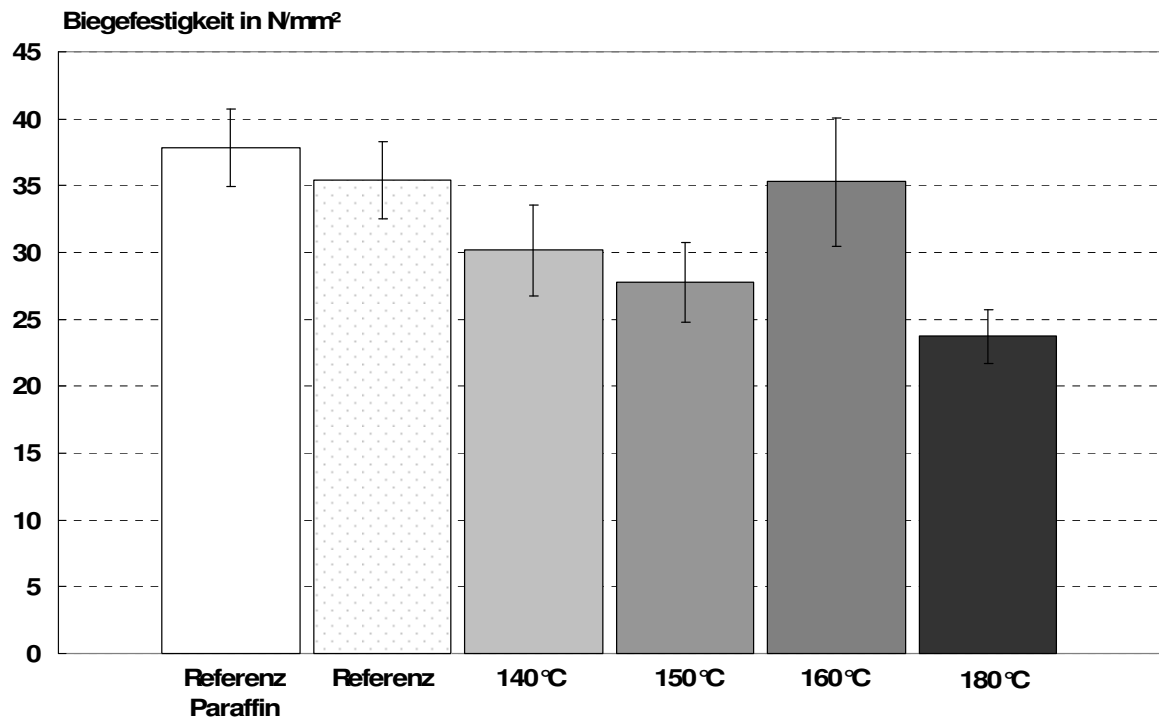
Abbildung 4: Biegefestigkeit PMDI-gebundener Kiefer-OSB, deren Strands bei 140°C bis 180°C thermisch modifiziert wurden.
