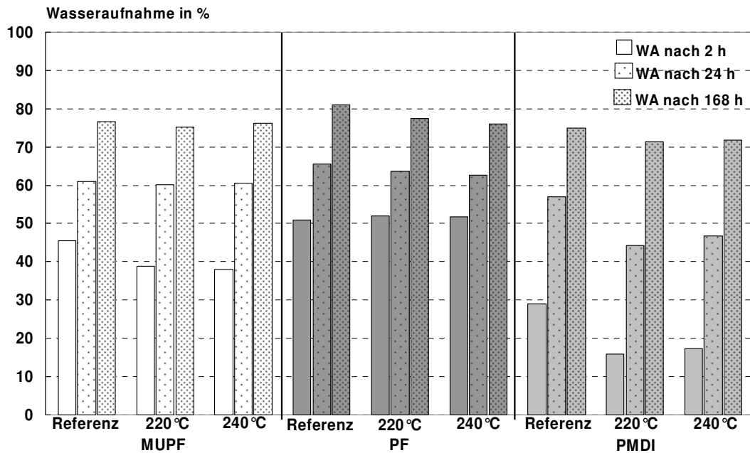
Abbildung 17: Wasseraufnahme (WA) nach 2, 24 und 168 Stunden Wasserlagerung von OSB aus Kiefer. Die bei 220°C und 240°C vorbehandelten Strands sowie unbehandelte Referenzstrands wurden mit MUPF, PF und PMDI zu Platten verpresst.
