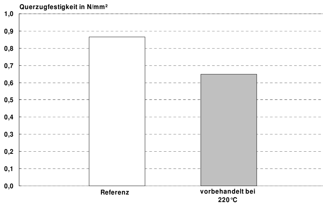
Abbildung 53: Querzugfestigkeit nach BAM-Zyklus von OSB aus Pappel. Die bei 220°C vorbehandelten Strands sowie unbehandelte Referenzstrands wurden mit PMDI zu Platten verpresst.
