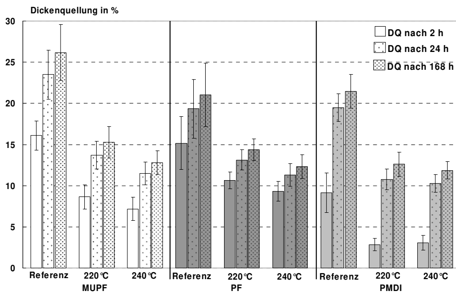
Abbildung 16: Dickenquellung (DQ) nach 2, 24 und 168 Stunden Wasserlagerung von OSB aus Kiefer. Die bei 220°C und 240°C vorbehandelten Strands sowie unbehandelte Referenzstrands wurden mit MUPF, PF und PMDI zu Platten verpresst.
