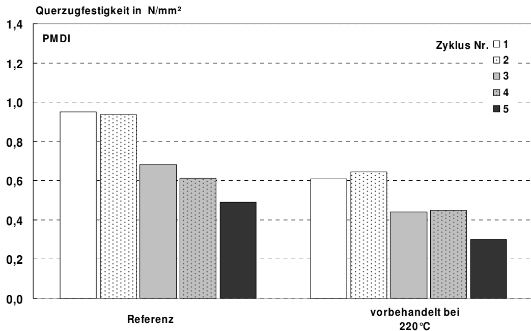
Abbildung 55: Querzugfestigkeit nach Zyklustest (2) von OSB aus Pappel. Die bei 220°C vorbehandelten Strands sowie unbehandelte Referenzstrands wurden mit PMDI zu Platten verpresst.
