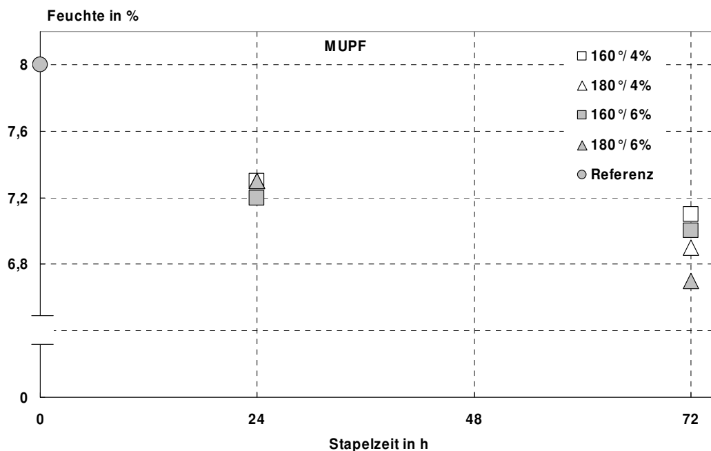
Abbildung 59: Gleichgewichtsfeuchte bei 20°C und 65% r. Lf. MUPF-gebundener OSB infolge Nachbehandlung im Stapel im Vergleich zur Referenz.
