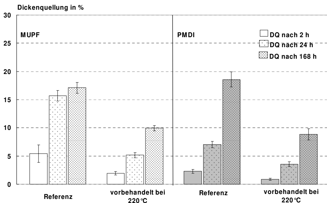
Abbildung 20: Dickenquellung (DQ) nach 2, 24 und 168 Stunden Wasserlagerung von Spanplatten aus Fichte. Die bei 220°C vorbehandelten Späne sowie unbehandelte Referenzspäne wurden mit MUPF und PMDI zu Platten verpresst.
