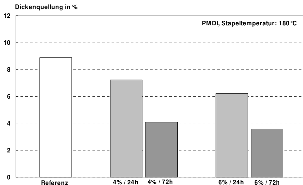
Abbildung 84: Irreversible Dickenquellung nach künstlicher Bewitterung und Klimatisierung bei 20°C und 65% r. Lf. von PMDI-gebundenen Platten, die bei 180°C für 24 bzw. 72 Stunden im Stapel nachbehandelt wurden; die Feuchte der Platten war auf 4% bzw. 6% eingestellt.
