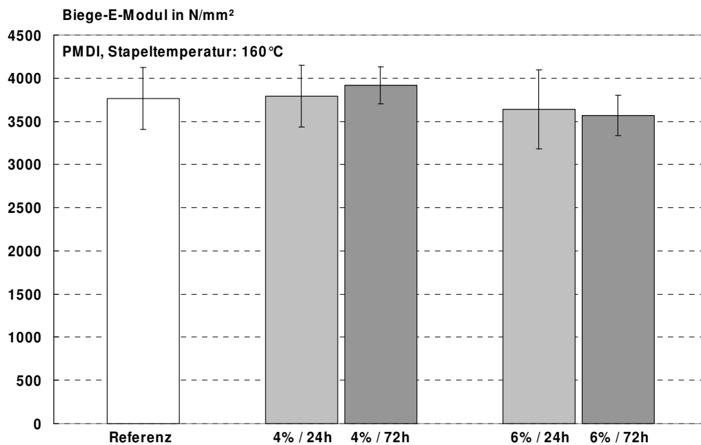
Abbildung 77: Biege-E-Modul von PMDI-gebundenen Platten, die bei 160°C für 24 bzw. 72 Stunden im Stapel nachbehandelt wurden; die Feuchte der Platten war auf 4% bzw. 6% eingestellt.
