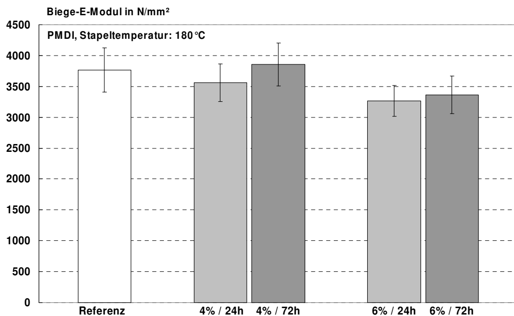
Abbildung 78: Biege-E-Modul von PMDI-gebundenen Platten, die bei 180°C für 24 bzw. 72 Stunden im Stapel nachbehandelt wurden; die Feuchte der Platten war auf 4% bzw. 6% eingestellt.
