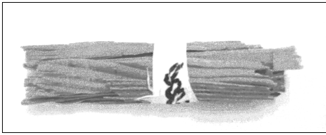
Abbildung 7: Mittels Teflonband gebündelte OSB-Strands aus Kiefer zur Prüfung der Dauerhaftigkeit nach EN 350.
