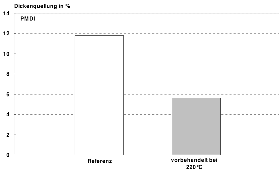
Abbildung 52: Irreversible Dickenquellung nach BAM-Zyklus von OSB aus Pappel. Die bei 220°C vorbehandelten Strands sowie unbehandelte Referenzstrands wurden mit PMDI zu Platten verpresst.
