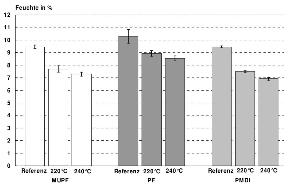
Abbildung 15: Gleichgewichtsfeuchte bei 20°C und 65% r. Lf.. von OSB aus Kiefer. Die bei 220°C und 240°C vorbehandelten Strands sowie unbehandelte Referenzstrands wurden mit MUPF, PF und PMDI zu Platten verpresst.
