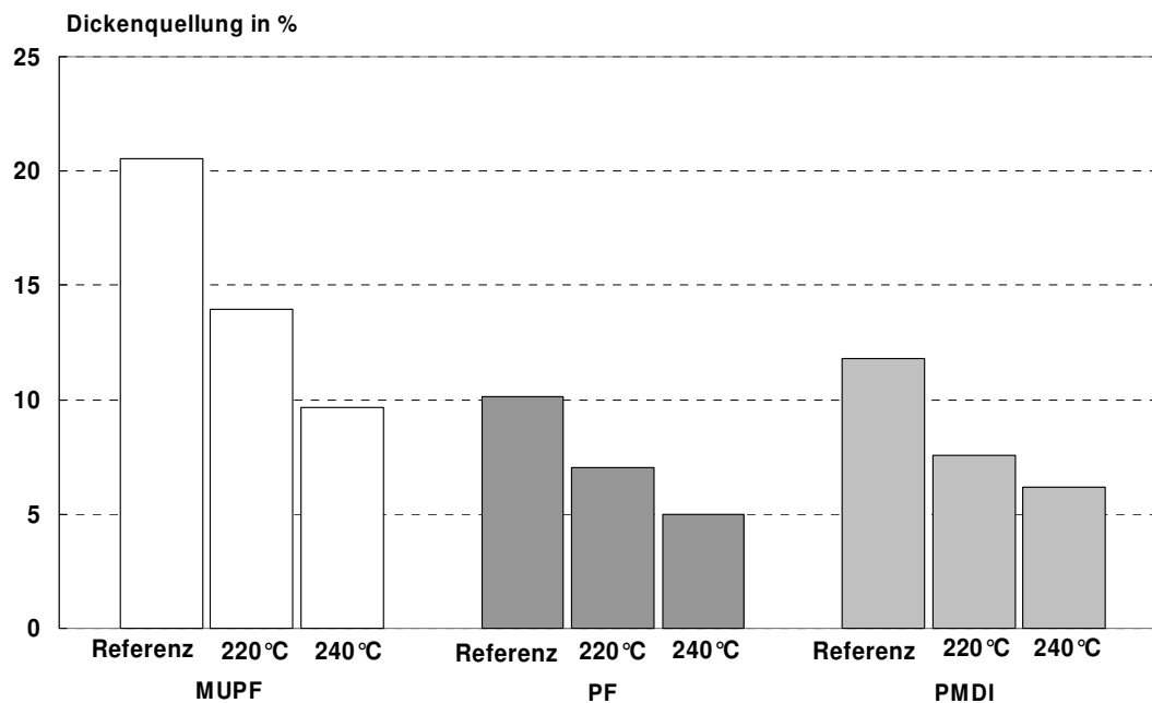
Abbildung 18: Irreversible Dickenquellung (IDQ) nach 168 Stunden Wasserlagerung von OSB aus Kiefer. Die bei 220°C und 240°C vorbehandelten Strands sowie unbehandelte Referenzstrands wurden mit MUPF, PF und PMDI zu Platten verpresst.
