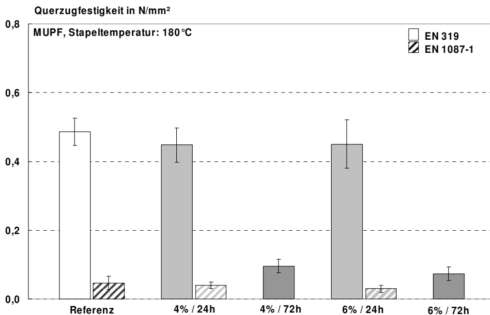
Abbildung 70: Querzugfestigkeit trocken (EN 319) sowie nach Kochtest (EN 1087-1) von MUPF-gebundenen Platten, die bei 180°C für 24 bzw. 72 Stunden im Stapel nachbehandelt wurden; die Feuchte der Platten war auf 4% bzw. 6% eingestellt.
