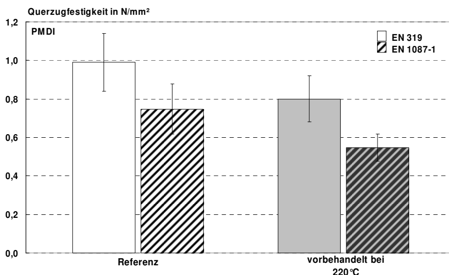
Abbildung 29: Querzugfestigkeit (QZ) trocken (EN 319) und nach Kochtest (EN 1087-1) von OSB aus Pappel. Die bei 220°C vorbehandelten Strands sowie unbehandelte Referenzstrands wurden mit PMDI zu Platten verpresst.
