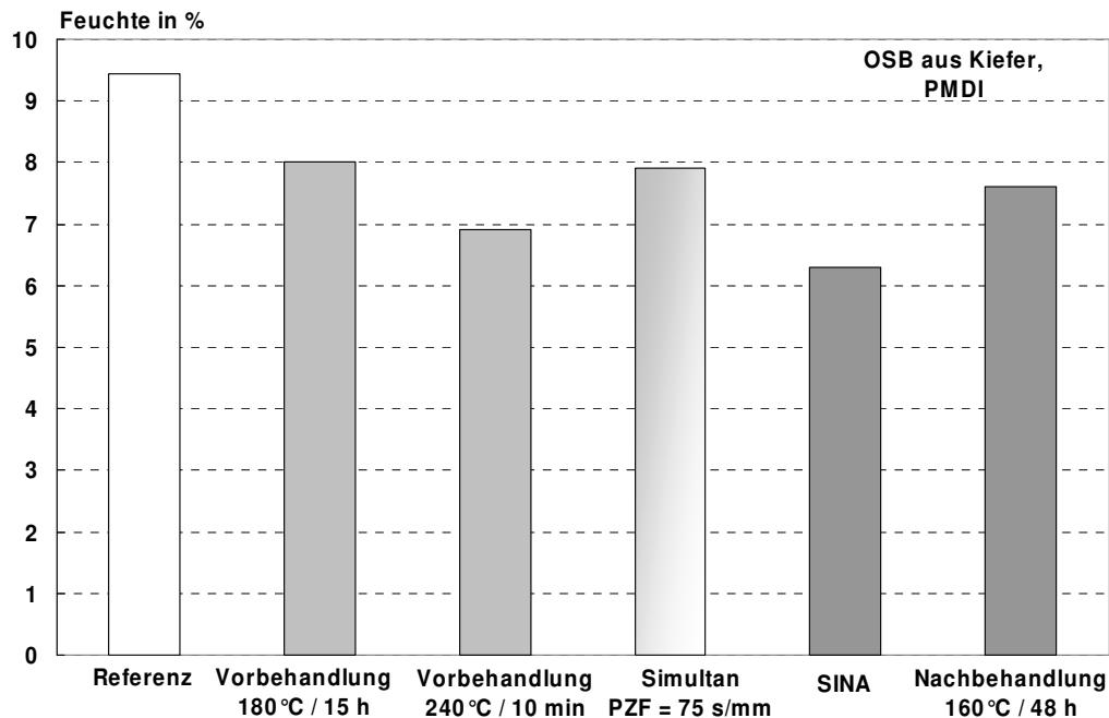
Abbildung 95: Gleichgewichtsfeuchte bei 20°C und 65% r. Lf. PMDI-gebundener OSB aus Kiefer, hergestellt nach verschiedenen Verfahren zur thermischen Modifizierung.
