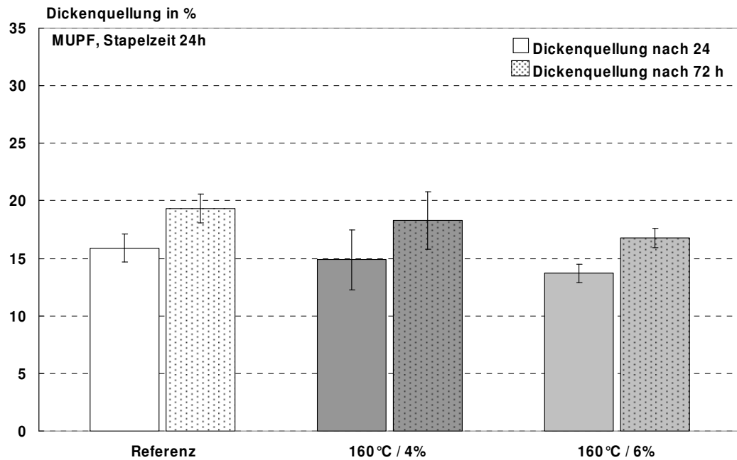
Abbildung 61: Dickenquellung nach 24 und 72 Stunden Wasserlagerung von MUPF-gebundenen Platten, die für 24 Stunden bei 160°C nachbehandelt wurden; die Feuchte der Platten war auf 4% bzw. 6% eingestellt.
