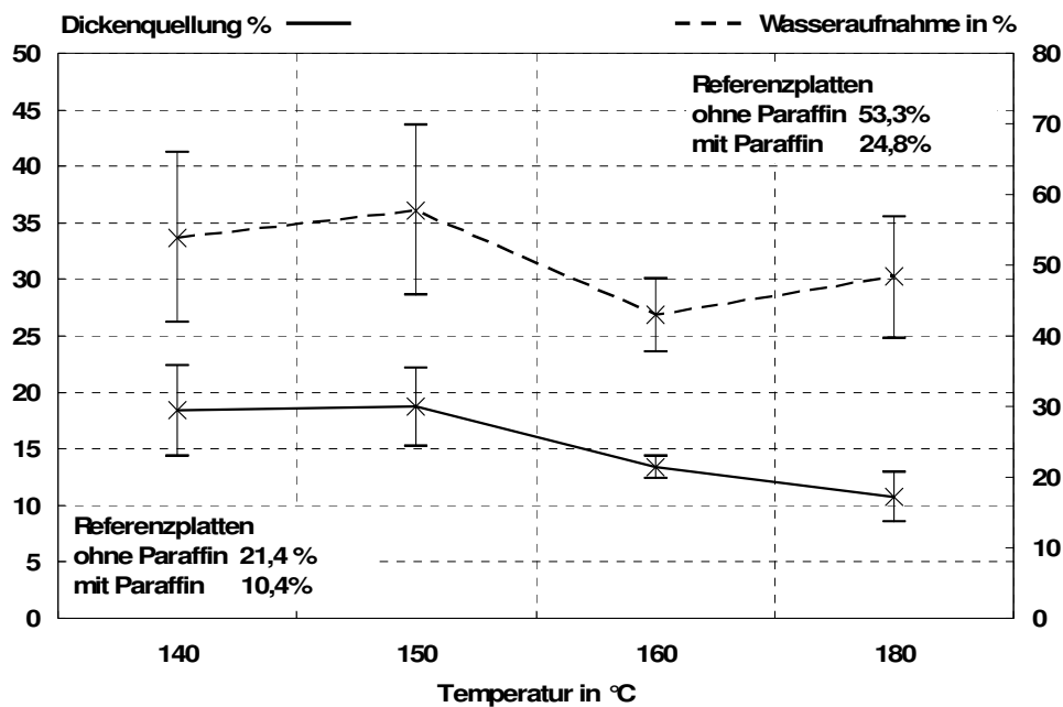
Abbildung 2: Dickenquellung und Wasseraufnahme nach 24 Stunden Wasserlagerung von OSB aus Kiefer, deren Strands bei 140°C bis 180°C in Luftatmosphäre vorbehandelt wurden.
