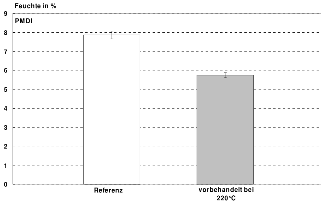
Abbildung 23: Gleichgewichtsfeuchte bei 20°C und 65% r. Lf. von OSB aus Pappel. Die bei 220°C vorbehandelten Strands sowie unbehandelte Strands wurden mit PMDI zu Platten verpresst.
