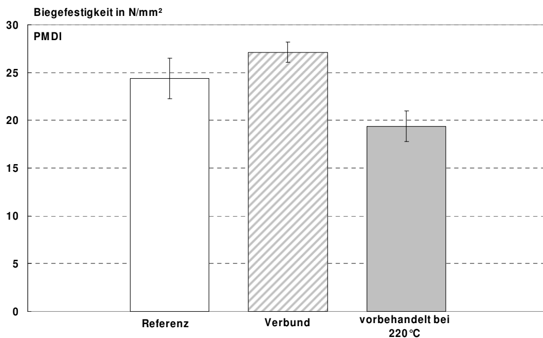
Abbildung 40: Biegefestigkeit PMDI-gebundener Fichtespanplatten aus unbehandelten und thermisch modifizierten Spänen sowie aus einem Verbund beider Spantypen.
