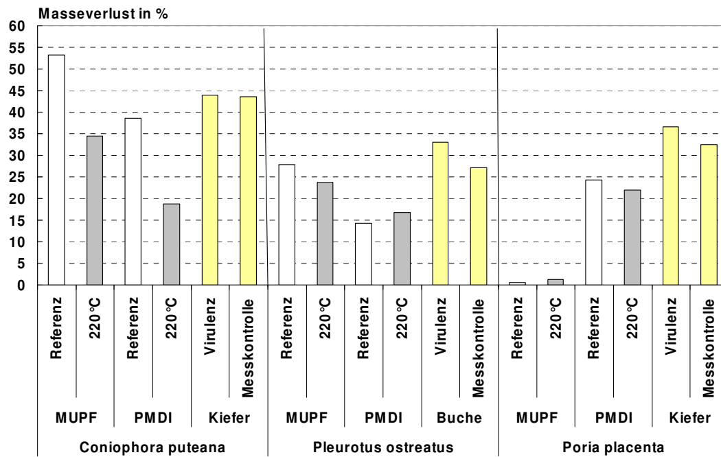
Abbildung 57: Masseverlust durch Coniophora puteana , Pleurotus ostreatus und Poria placenta nach 16wöchiger Inkubationszeit von Spanplatten aus Fichte. Die bei 220°C vorbehandelten Späne sowie unbehandelte Referenzspäne wurden mit MUPF und PMDI zu Platten verpresst.
