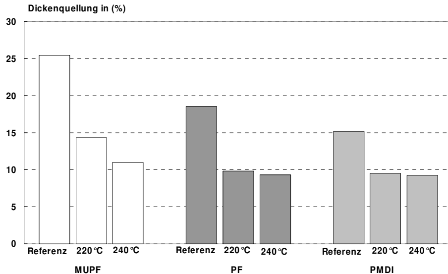
Abbildung 44: Irreversible Dickenquellung nach BAM-Zyklus von OSB aus Kiefer. Die bei 220^\circ\text{C} und 240^\circ\text{C} behandelten Strands sowie unbehandelte Referenzstrands wurden mit MUPF, PF und PMDI zu Platten verpresst.
