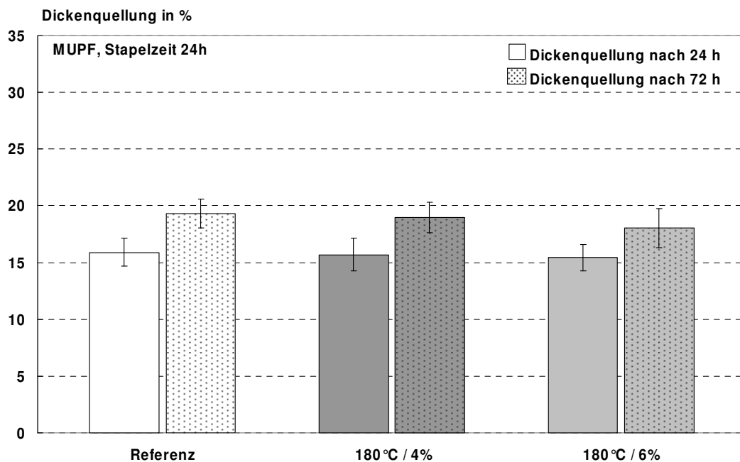
Abbildung 62: Dickenquellung nach 24 und 72 Stunden Wasserlagerung von MUPF-gebundenen Platten, die für 24 Stunden bei 180°C nachbehandelt wurden; die Feuchte der Platten war auf 4% bzw. 6% eingestellt.
