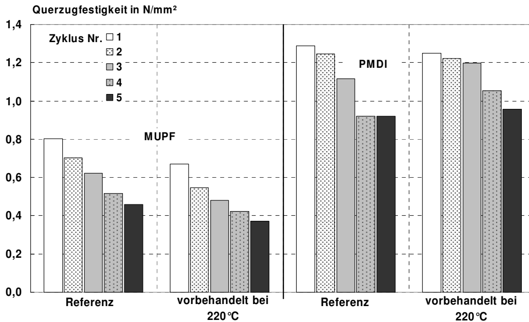
Abbildung 51: Querzugfestigkeit nach Zyklustest (2) von Spanplatten aus Fichte. Die bei 220°C vorbehandelten Späne sowie unbehandelte Referenzspäne wurden mit MUPF und PMDI zu Platten verpresst.
