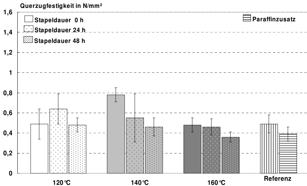
Abbildung 92: Querzugfestigkeit nach Kochtest (EN 1087-1) von OSB, die bei 120°C, 140°C bzw. 160°C für 24 bzw. 48 Stunden im Stapel nachbehandelt wurden im Vergleich zur Referenz. Die Presszeit hing von der angestrebten Stapeltemperatur ab (Stapeldauer 0 h).
