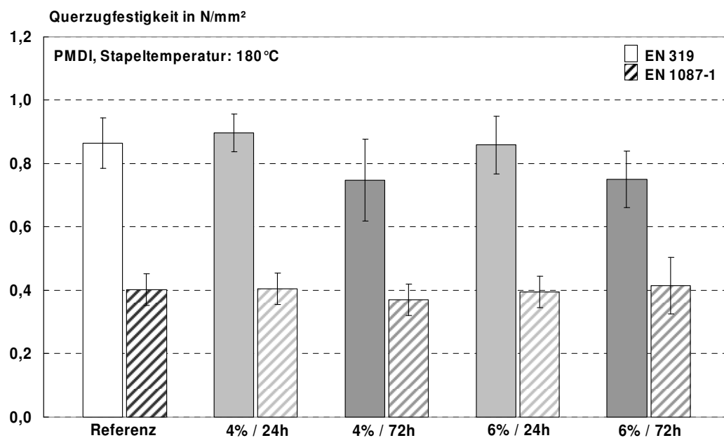
Abbildung 72: Querzugfestigkeit trocken (EN 319) sowie nach Kochtest (EN 1087-1) von PMDI-gebundenen Platten, die bei 180°C für 24 bzw. 72 Stunden im Stapel nachbehandelt wurden; die Feuchte der Platten war auf 4% bzw. 6% eingestellt.
