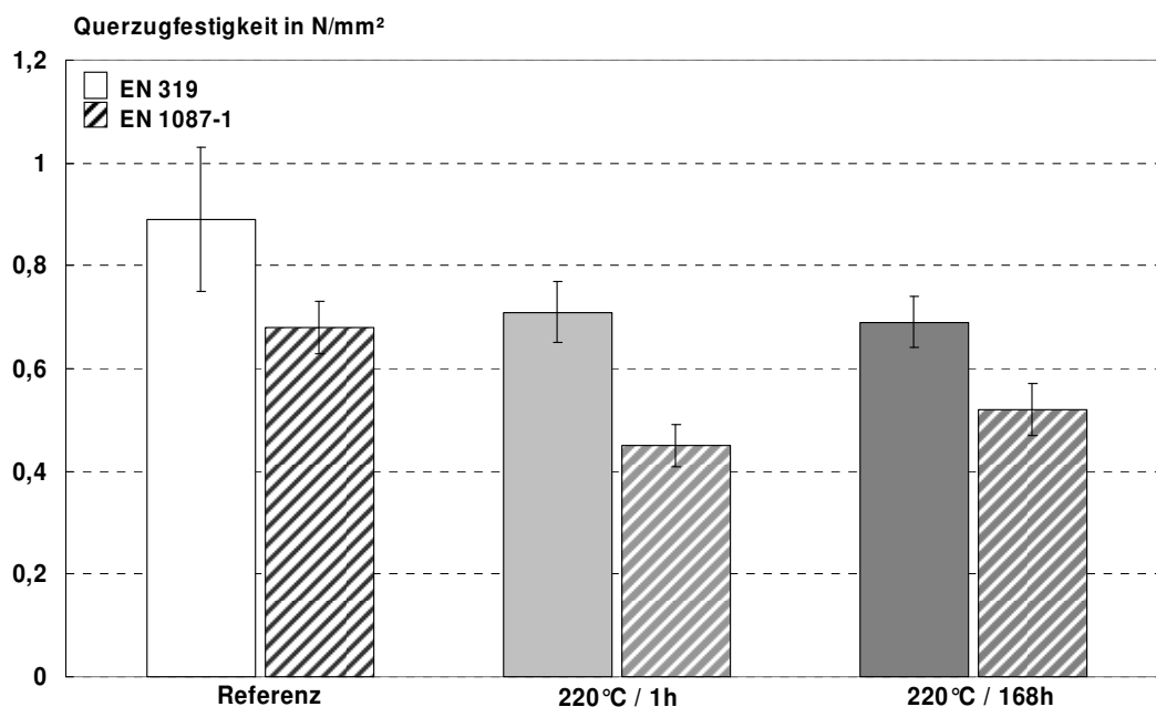
Abbildung 30: Querkzugfestigkeit trocken (EN 319) sowie nach Kochtest (EN 1087-1) von Kiefernspanplatten aus modifizierten Spänen im Vergleich zur unbehandelten Referenz. Die Platten aus vorbehandelten Spänen wurden 1 bzw. 168 Stunden nach der Vorbehandlung mit PF zu Platten verpresst.
