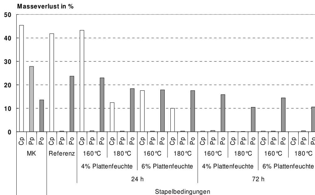
Abbildung 87: Masseverlust durch Coniophora puteana (Cp), Pleurotus ostreatus (Po) und Poria placenta (Pp) nach 16wöchiger Inkubationszeit von MUPF-gebundenen OSB aus Kiefer. Die Platten einer Feuchte von 4% bzw. 6% wurden durch Nachbehandlung im Stapel bei 160°C bzw. 180°C für 24 und 72 Stunden modifiziert.
