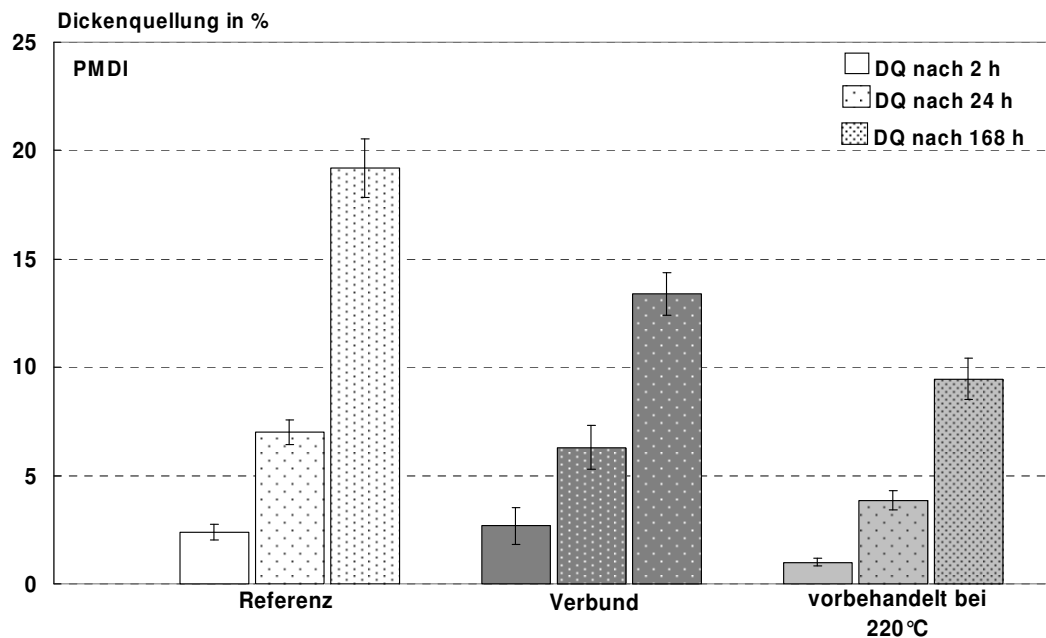
Abbildung 43: Dickenquellung nach zwei, 24 und 168 Stunden Wasserlagerung PMDI-gebundener Fichtespanplatten aus unbehandelten und thermisch modifizierten Spänen sowie einem Verbund aus beiden Spantypen.
