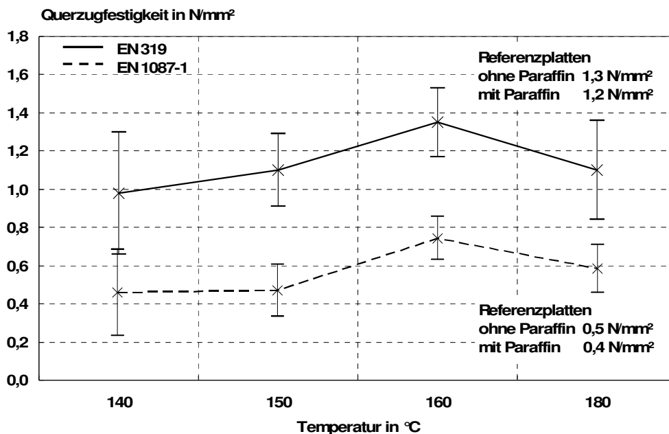
Abbildung 3: Querkzugfestigkeit vor (EN 319) und nach Kochtest (EN 1087-1) PMDI-gebundener Kiefer-OSB, deren Strands bei 140°C bis 180°C thermisch modifiziert wurden.
