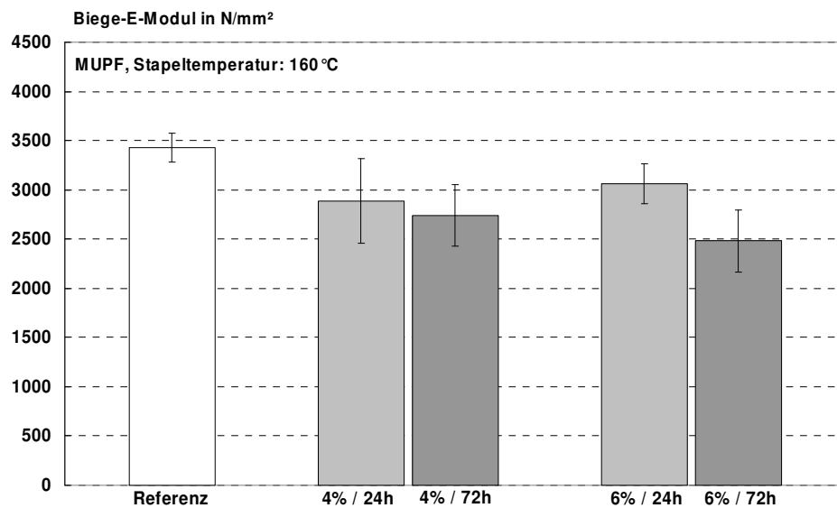
Abbildung 73: Biege-E-Modul von MUPF-gebundenen Platten, die bei 160°C für 24 bzw. 72 Stunden im Stapel nachbehandelt wurden; die Feuchte der Platten war auf 4% bzw. 6% eingestellt.
