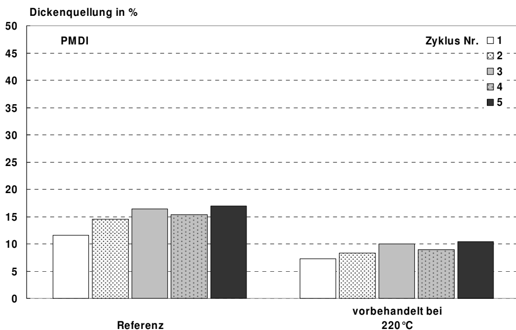
Abbildung 54: Irreversible Dickenquellung nach Zyklustest (2) von OSB aus Pappel. Die bei 220°C vorbehandelten Strands sowie unbehandelte Referenzstrands wurden mit PMDI zu Platten verpresst.
