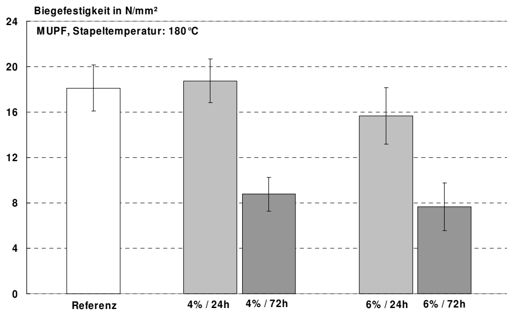
Abbildung 76: Biegefestigkeit von MUPF-gebundenen Platten, die bei 180°C für 24 bzw. 72 Stunden im Stapel nachbehandelt wurden; die Feuchte der Platten war auf 4% bzw. 6% eingestellt.
