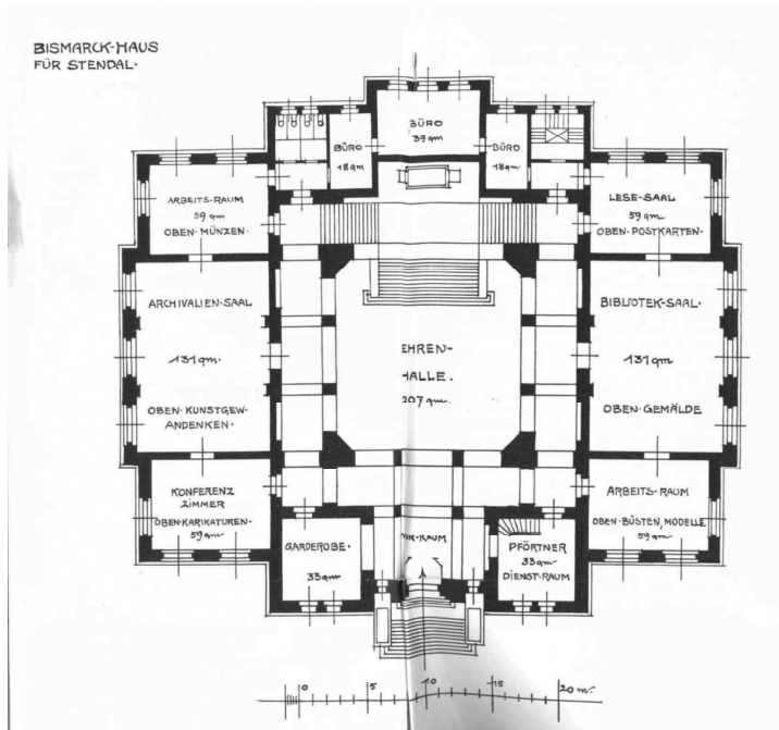
Abbildung 7: Grundriss des geplanten Bismarck-Hauses.
